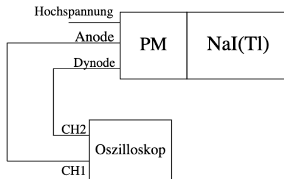
Abbildung 5.1: Schaltplan zur Kontrolle der Fast Pulse
