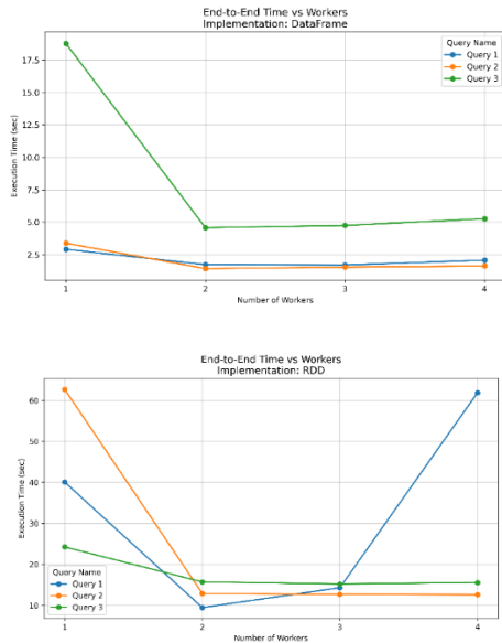
Figura 7. Confronto dei tempi End-to-end (Dataframe vs RDD)
