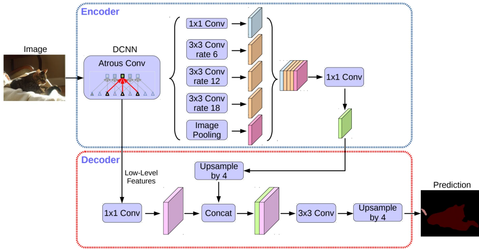
图 2-1 DeepLabV3+ 网络结构图 [7]
