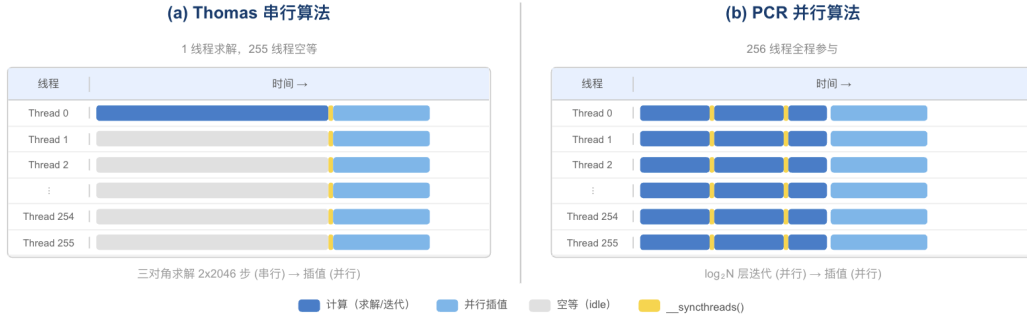
图 3-2 Thomas 算法与 PCR 算法的线程利用对比
