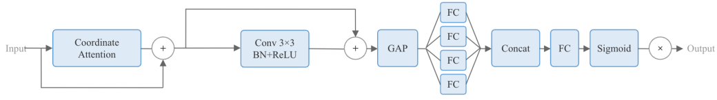
图 4-5 SAE 模块结构图
