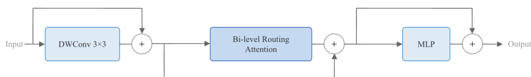
图 4-3 TR 模块结构图（窗口大小 S=4 ，窗口数量 S^2=16 ， \text{TopK}=4 ）
