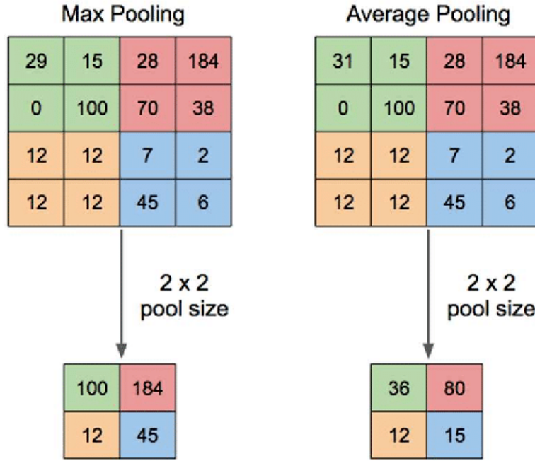
图 2-2 池化运算示意图 [55]
