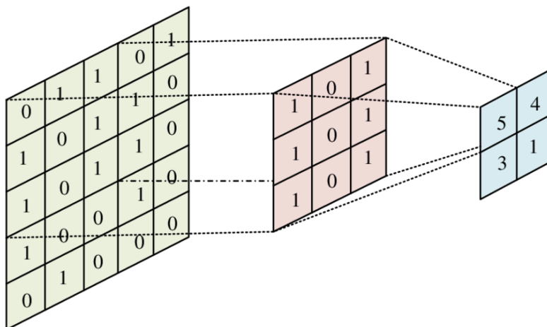
图 2-1 卷积运算示意图 [54]
