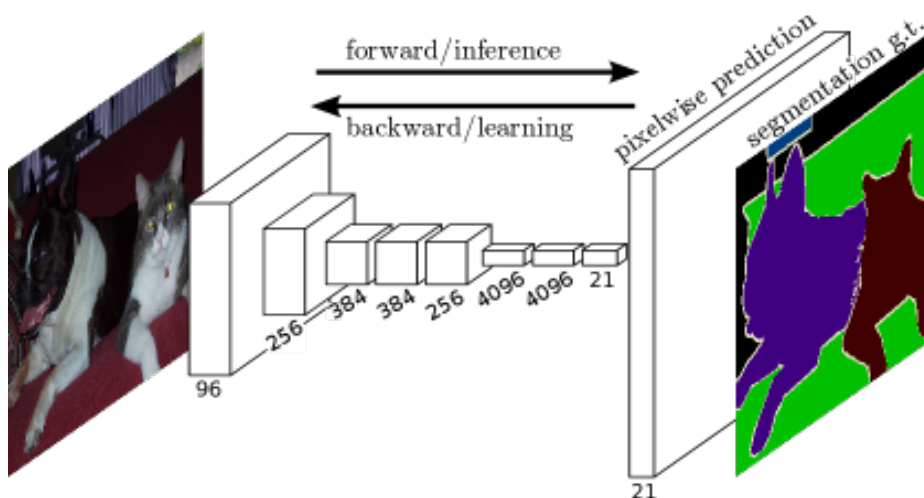
图 2-3 FCN 网络结构图 [5]
