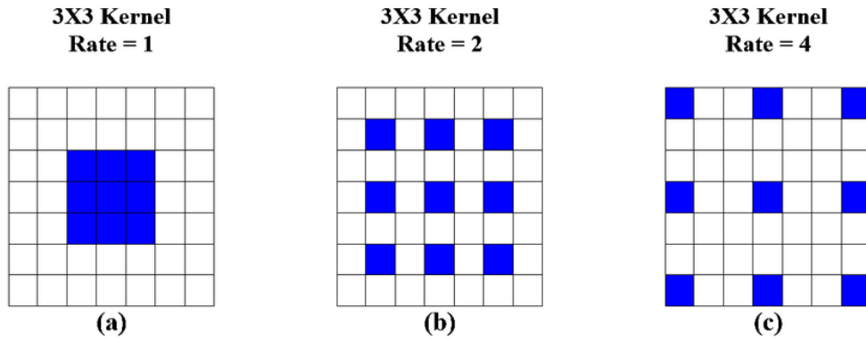
图 3-1 空洞卷积示意图 [62]
