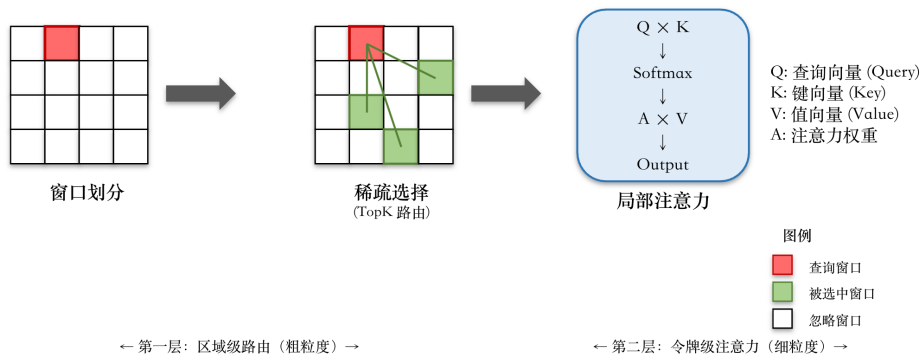
图 4-4 双层路由注意力机制示意图（窗口大小：4×4，窗口数量：16，TopK=4）
