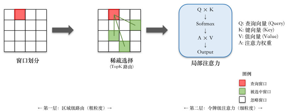
图 3-4 双层路由注意力机制示意图
