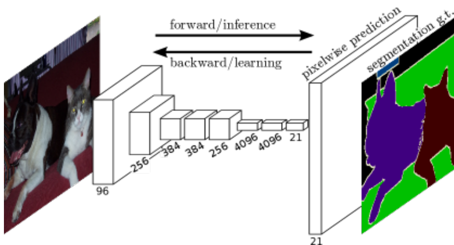
图 2-3 FCN 网络结构图 [3]
