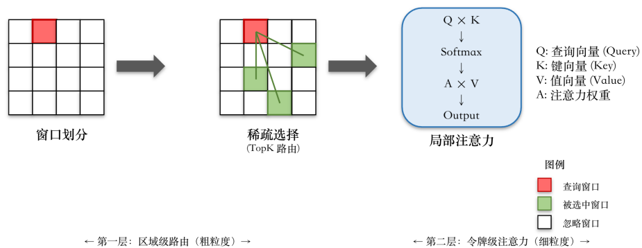
图 3-4 双层路由注意力机制示意图
