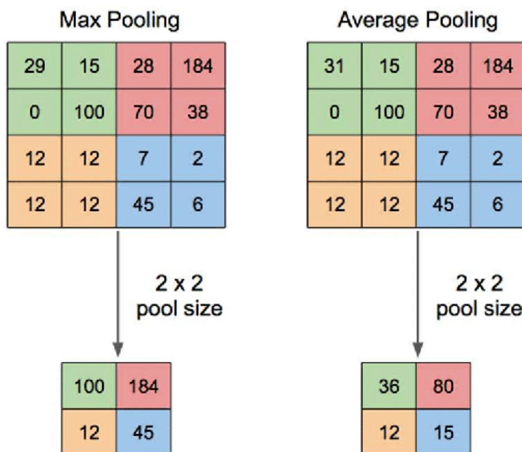
图 2-2 池化运算示意图 [54]
