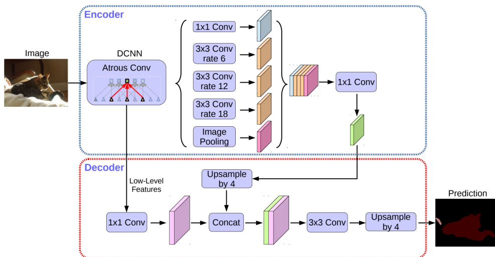
图 2-5 DeepLabV3+ 网络结构图 [5]
