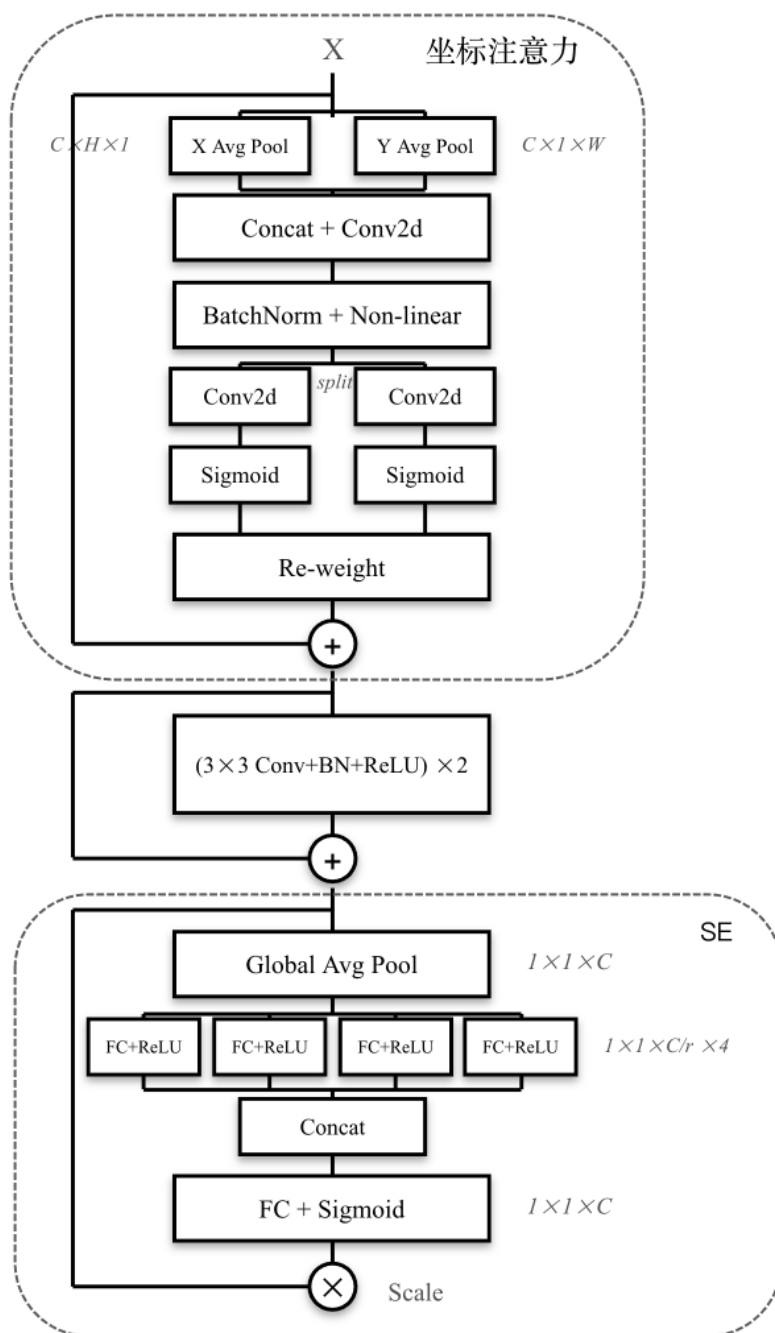
图 4-1 SAE 模块结构图
