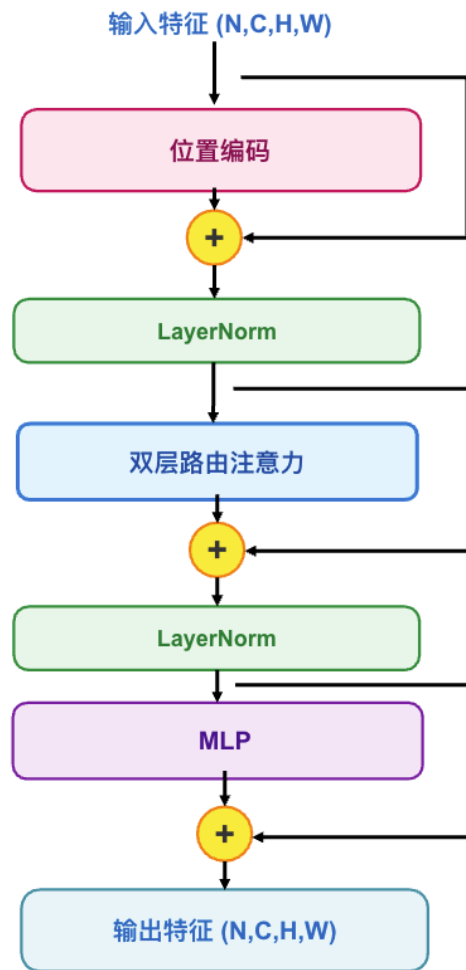
图 3-3 TR 模块结构图
