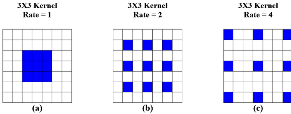
图 3-1 空洞卷积示意图 [63]
