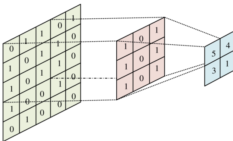
图 2-1 卷积运算示意图 [53]
