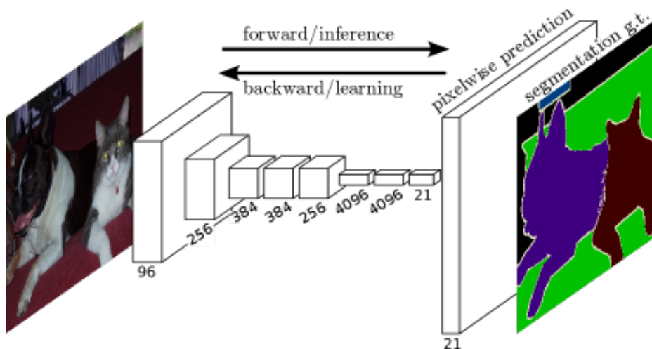
图 2-3 FCN 网络结构图 [3]
