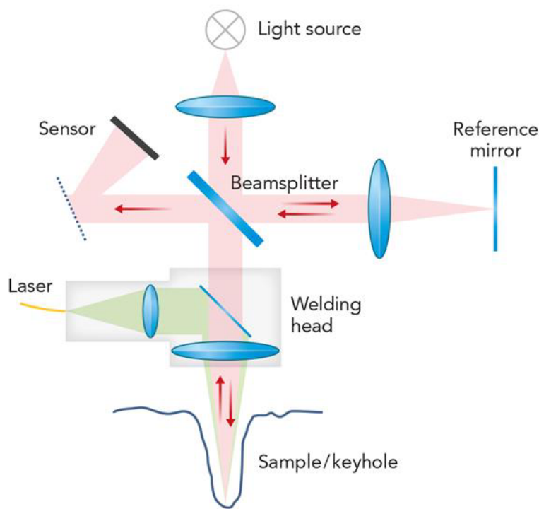
图 1-2 典型激光焊接过程监测系统示意图 [10]
