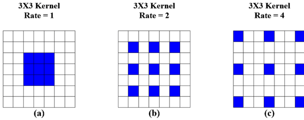
图 3-1 空洞卷积示意图 [66]
