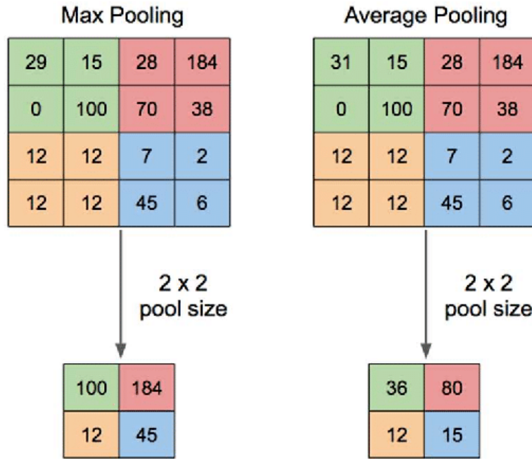
图 2-2 池化运算示意图 [57]
