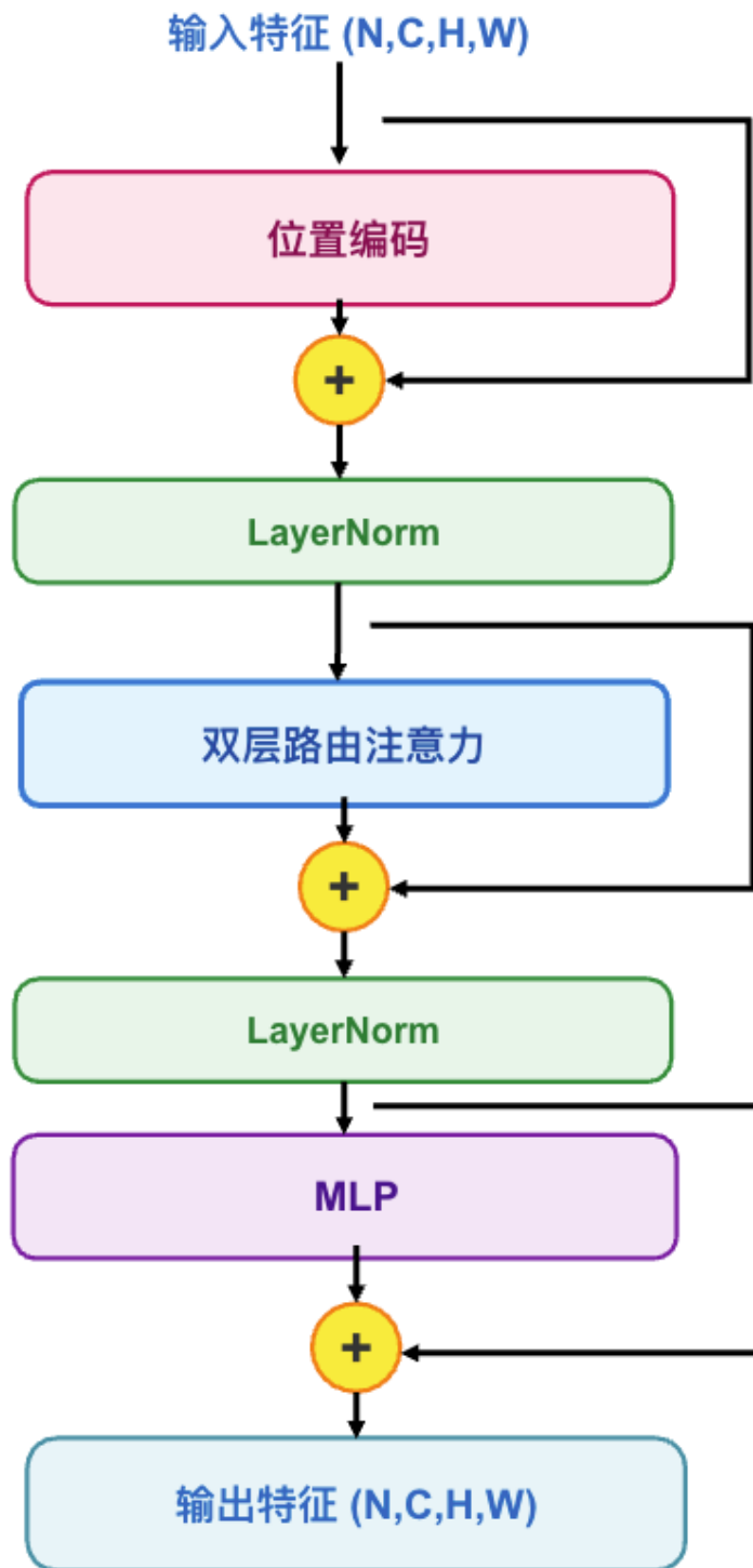
图 3-3 TR 模块结构图（输入：16×16×2560，输出：16×16×2560）
