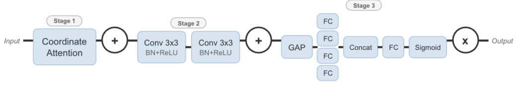
图 4-5 SAE 模块结构图（输入通道 C=560 ，Reduction r=4 ）
