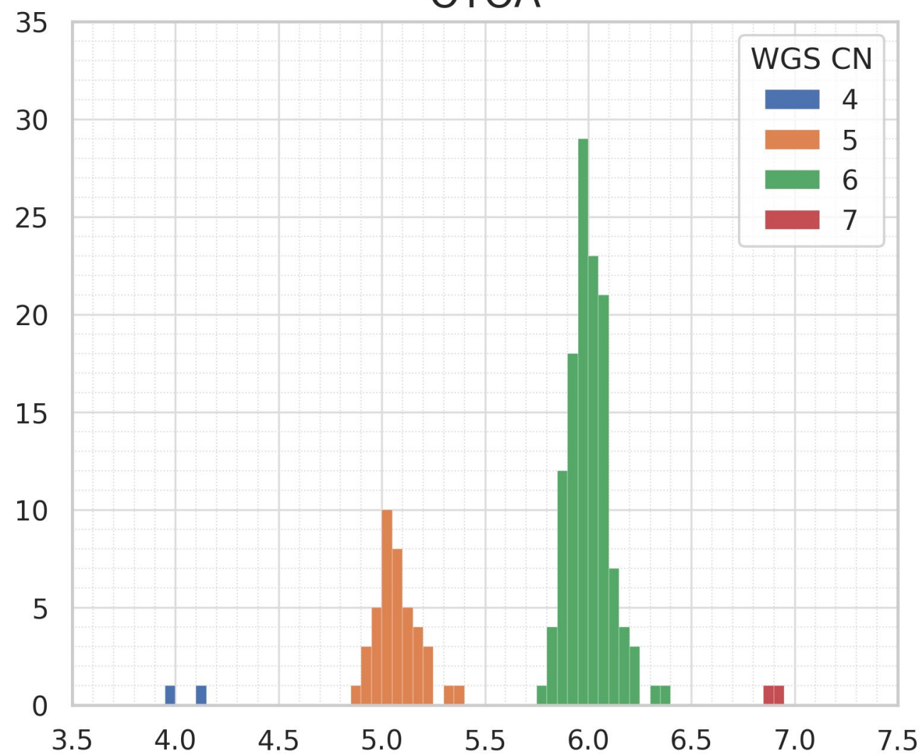
OTOA
