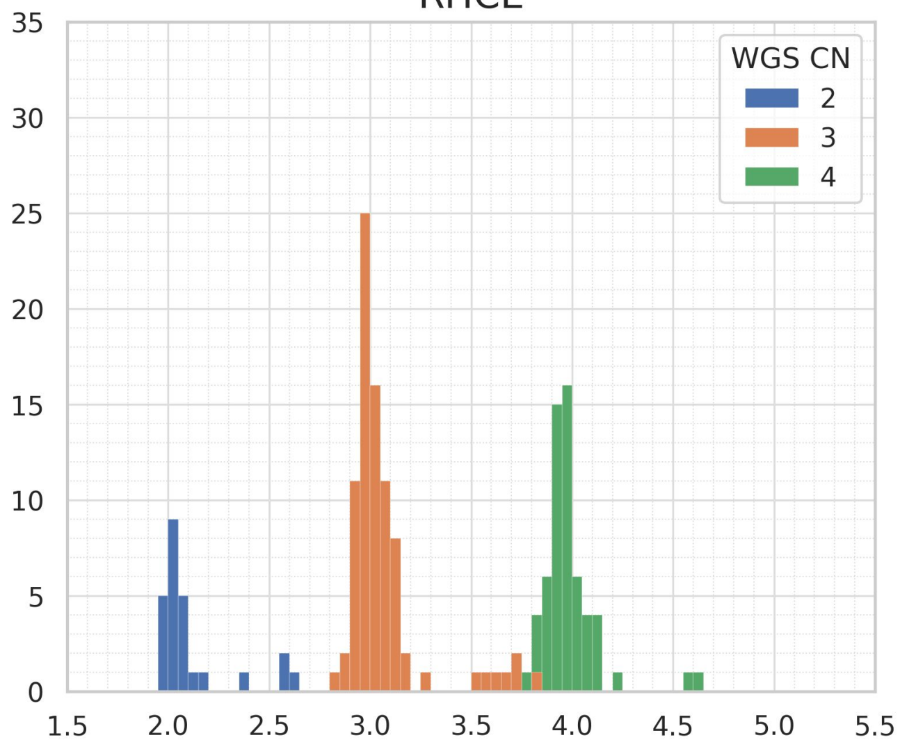
RHCE
