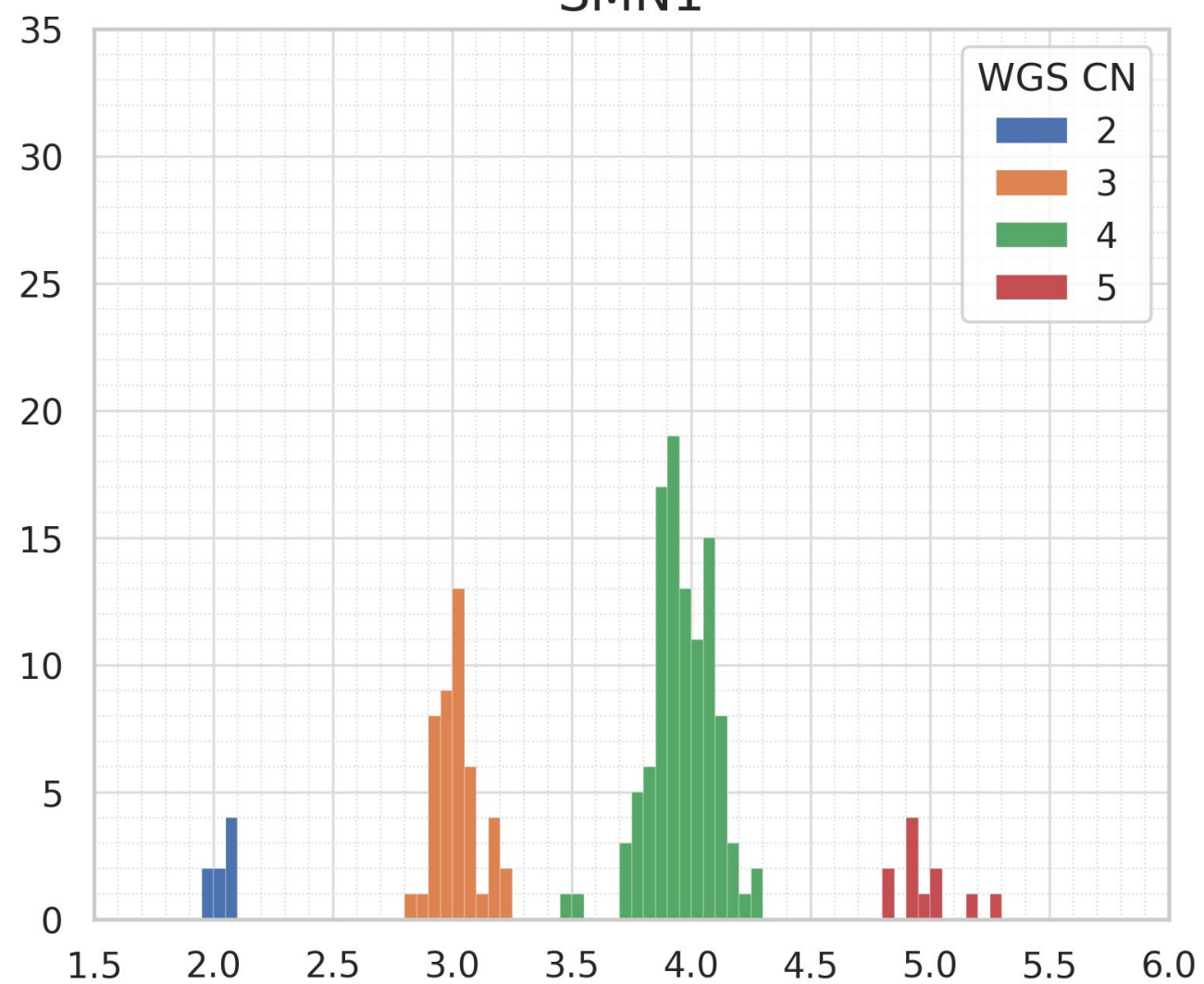
SMN1
