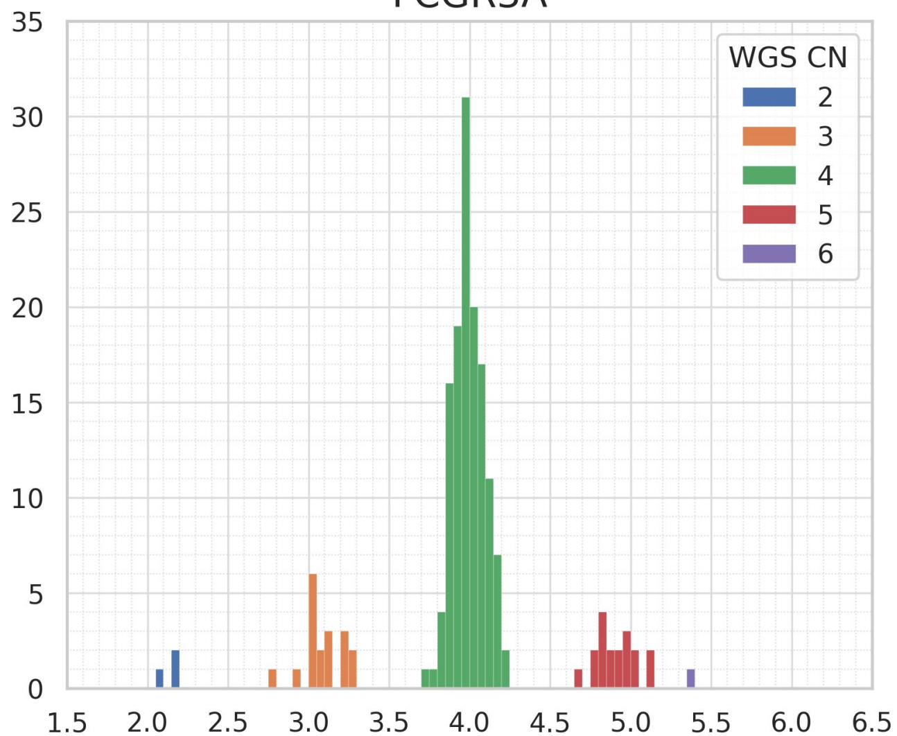
FCGR3A
