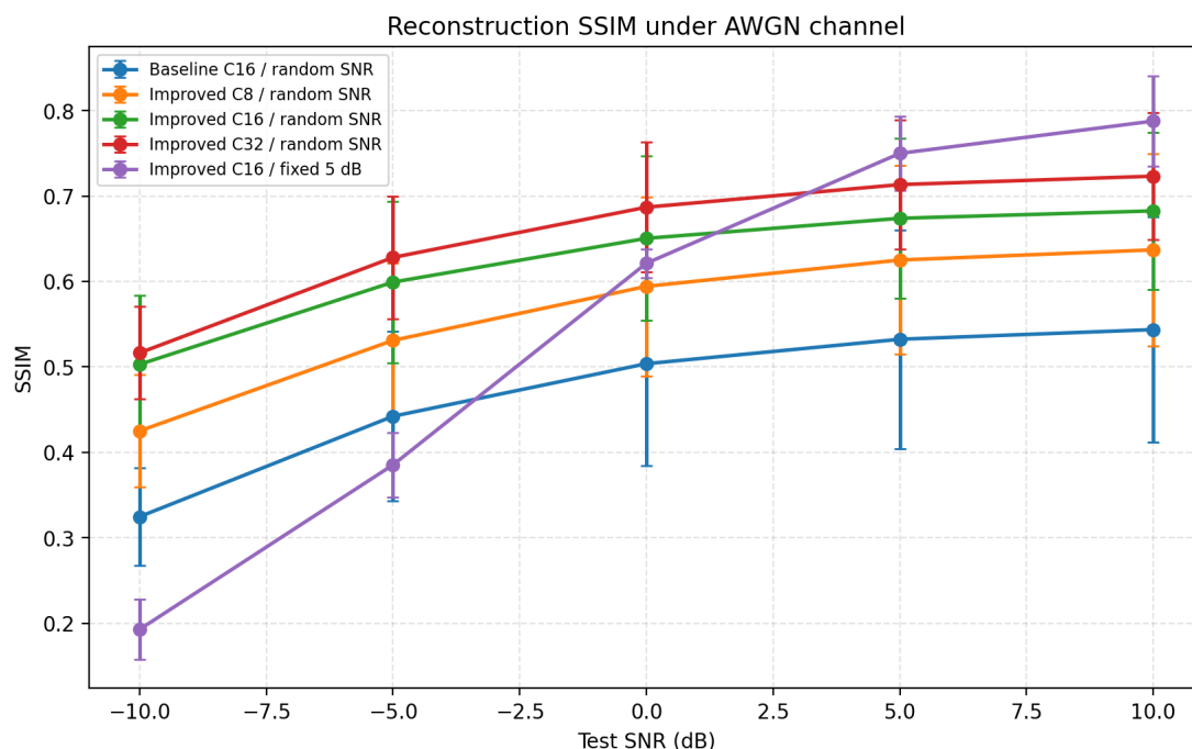
图5 不同 SNR 下的 SSIM 曲线
