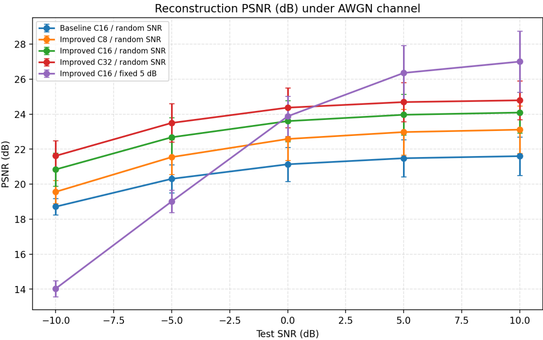
图4 不同 SNR 下的 PSNR 曲线
