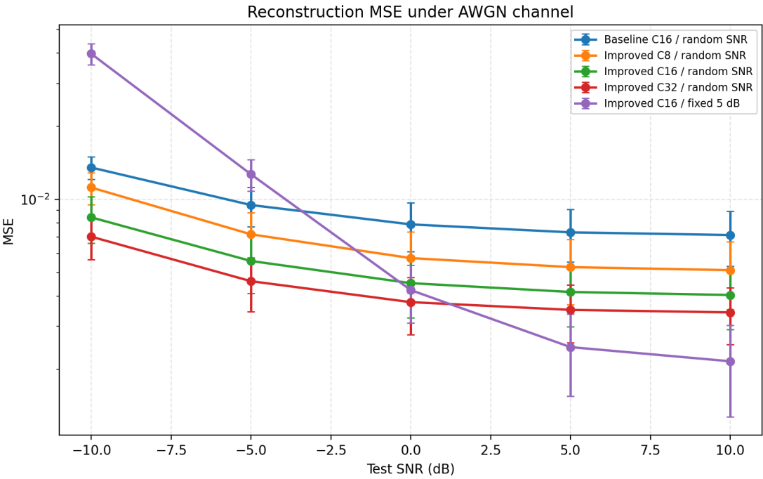
图3 不同 SNR 下的 MSE 曲线
