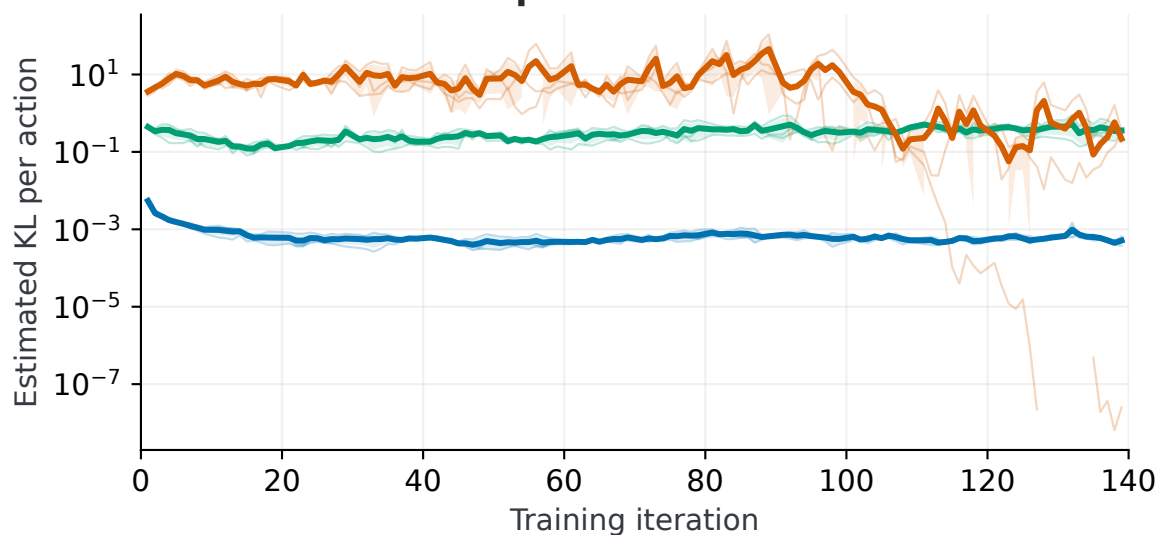
Post-update KL estimate
