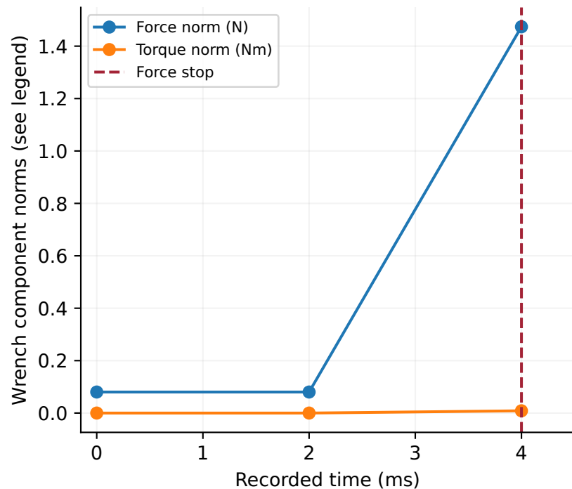
IMP99
