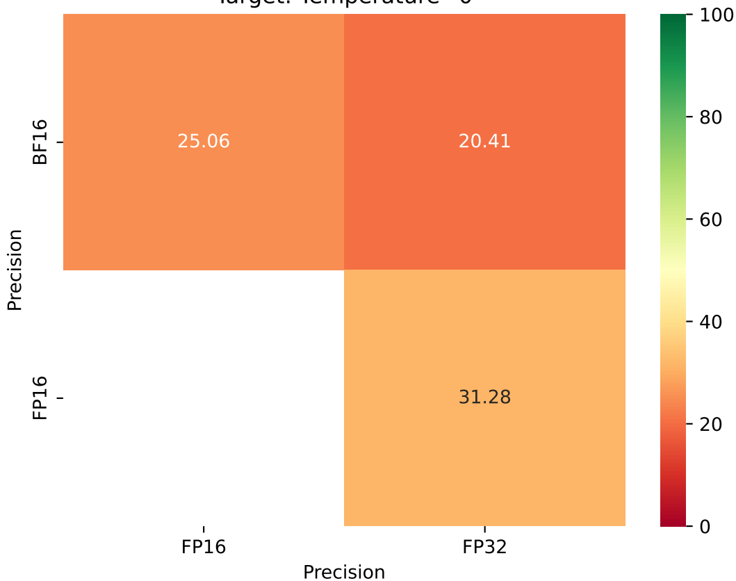
Llama-3.2-3B - Precision Consistency (%) Target: Temperature=0
