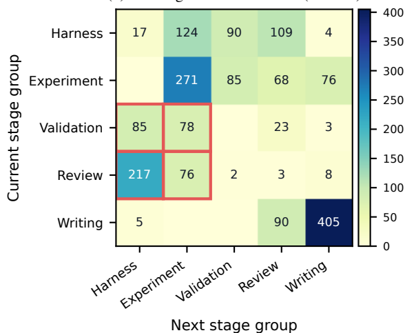
(d) Full stage-transition matrix (n=1853)
