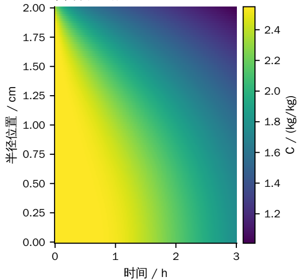
(b) 含水率场
