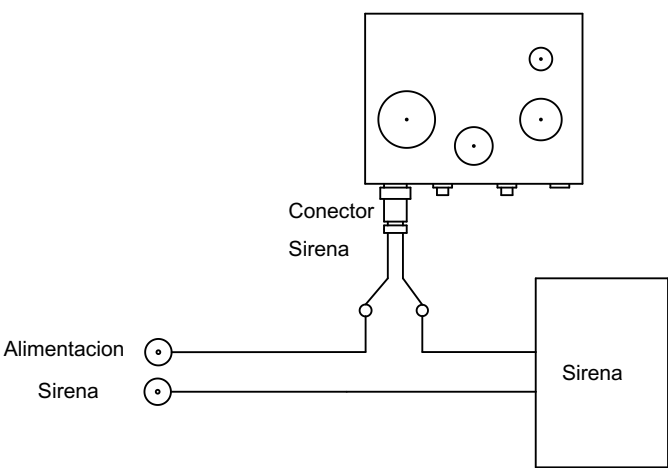
Esquema de sustitucion del pulsador por el temporizador
