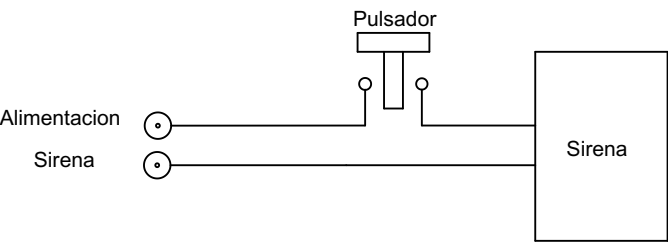
Esquema de sirena activada manualmente con un pulsador
