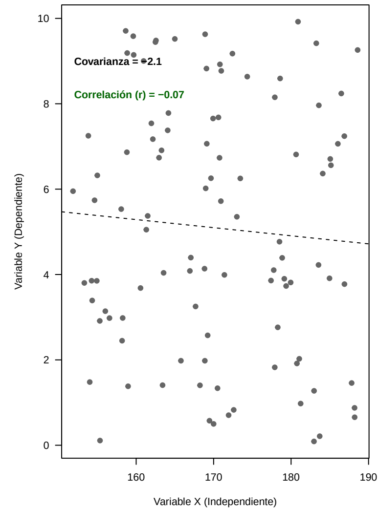
Sin Relación Lineal (Nula)
