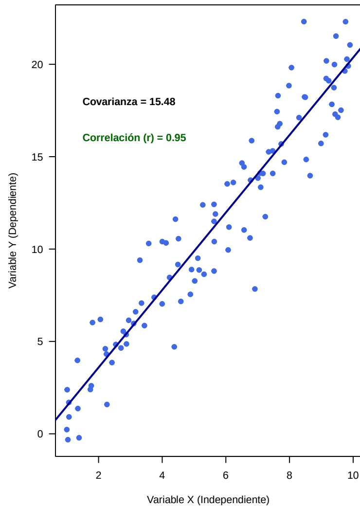
Relación Lineal Positiva
