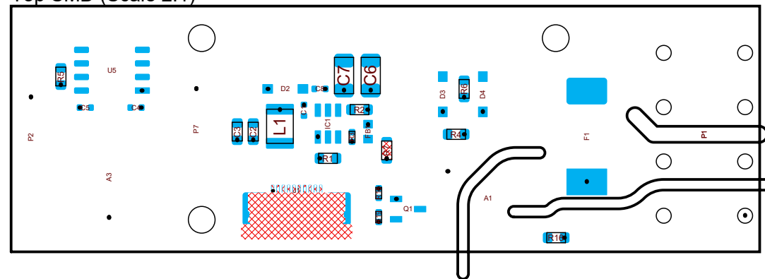
Top SMD (Scale 2:1)
