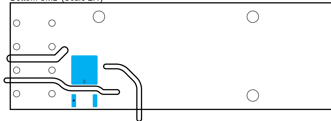
Bottom SMD (Scale 2:1)
