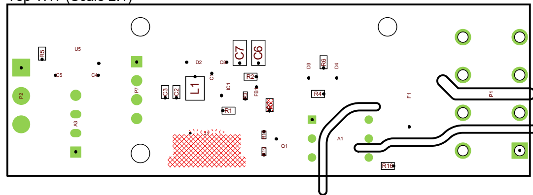
Top THT (Scale 2:1)
