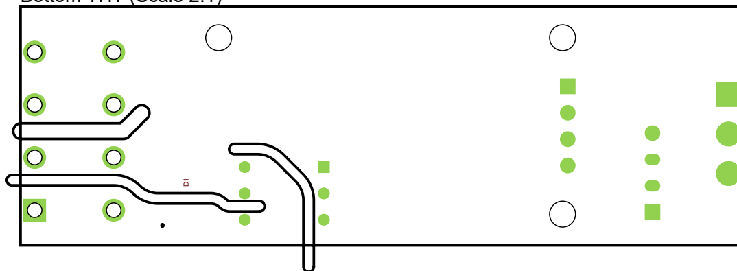
Bottom THT (Scale 2:1)
