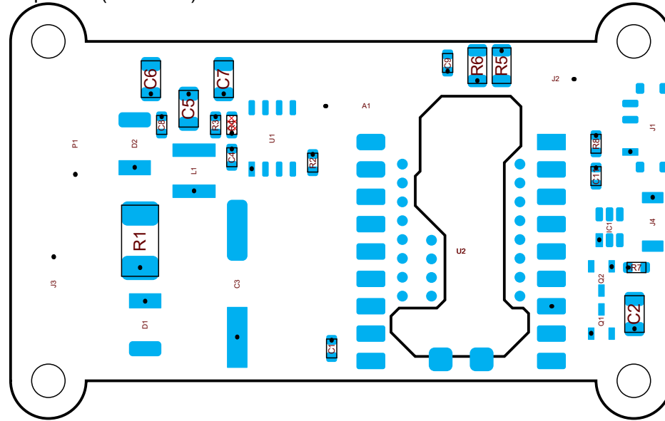
Top SMD (Scale 2:1)
