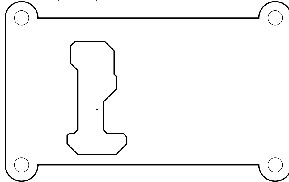
Bottom SMD (Scale 2:1)
