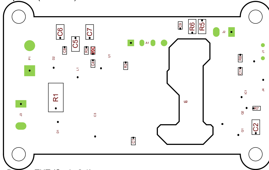
Bottom THT (Scale 2:1)
