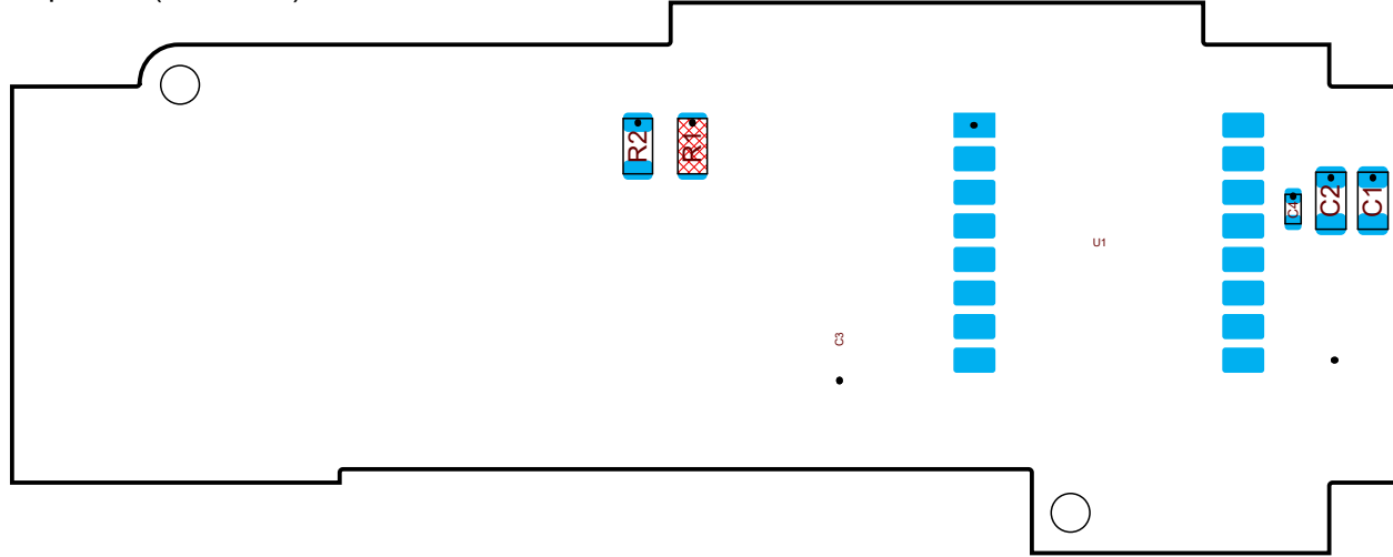
Top SMD (Scale 2:1)
