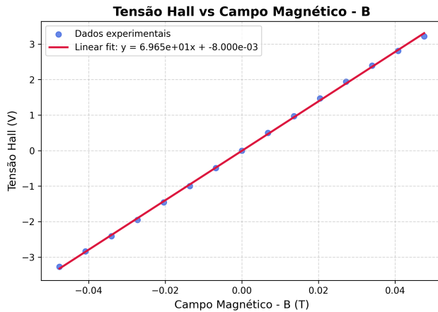
Figure 4: Tensão versos Campo
