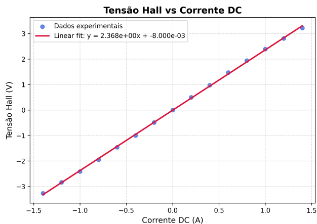
Figure 3: Tensão versus Corrente
