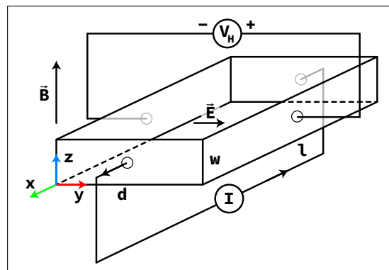
Figure 2: Diagrama dos campos
