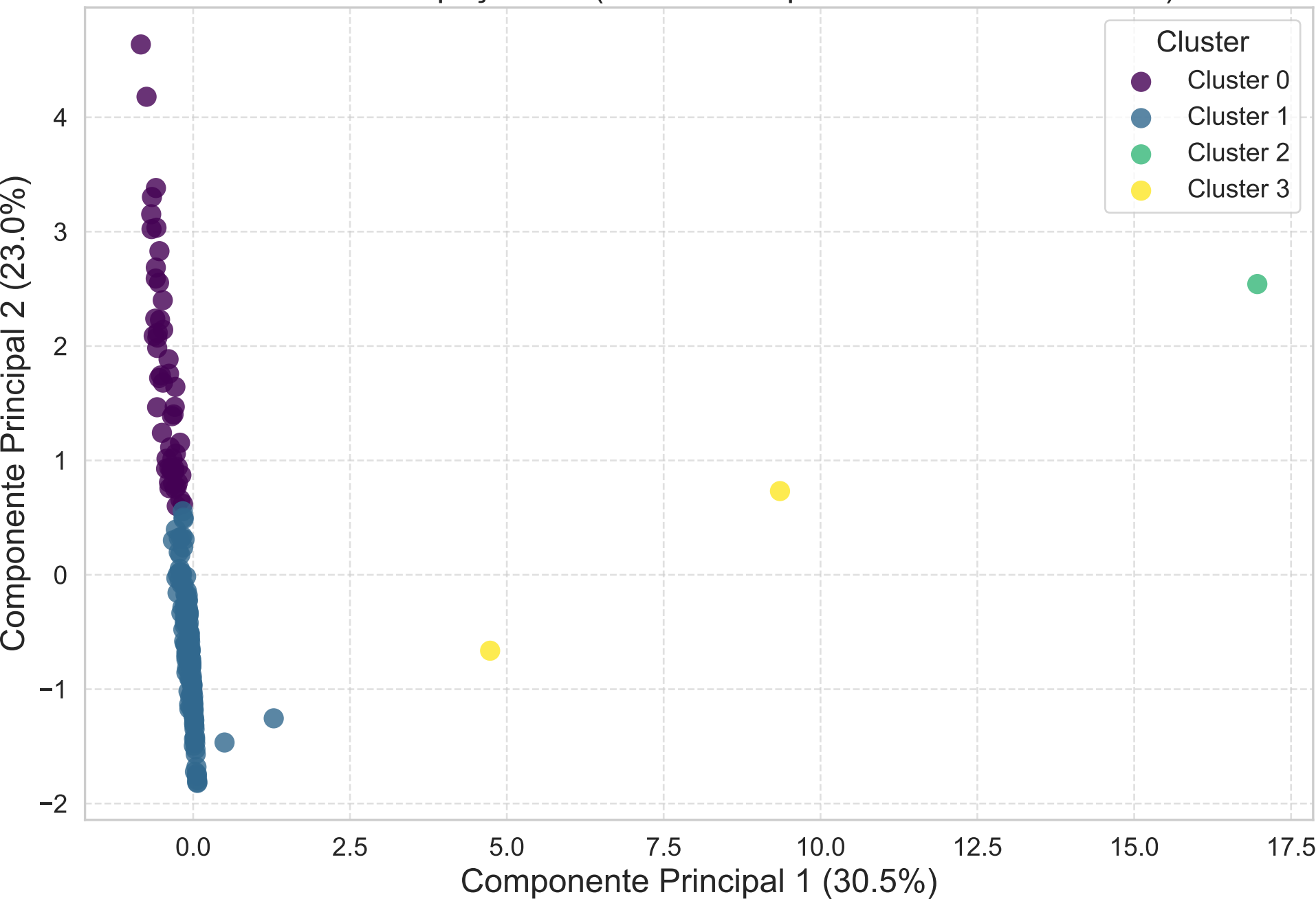
Clusters no Espaço PCA (Total Var. Explicada nos 2 PCs: 53.5%)
