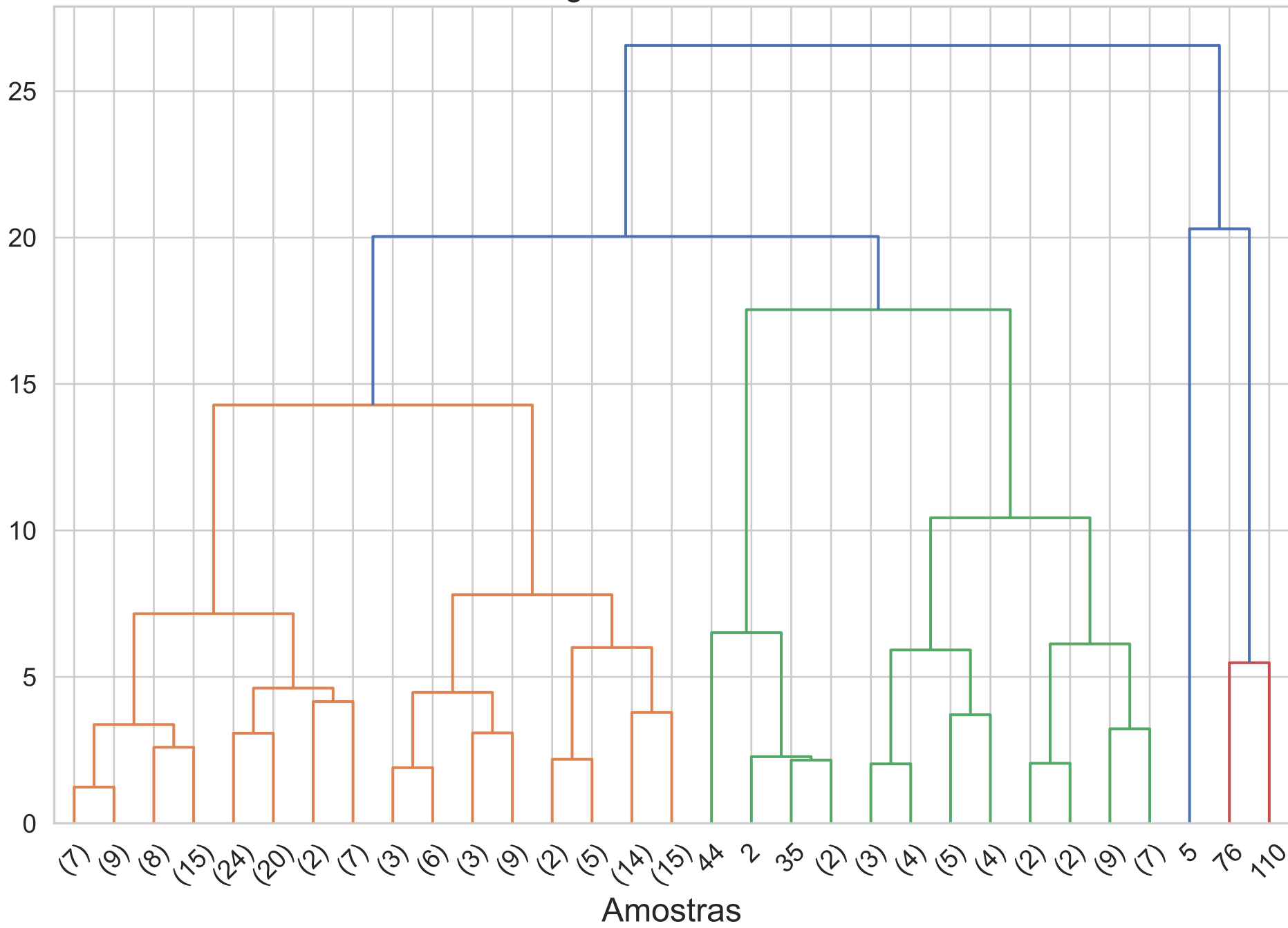
Dendrograma - Método Ward
