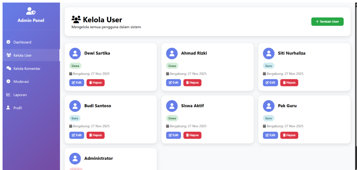
Kelola User
