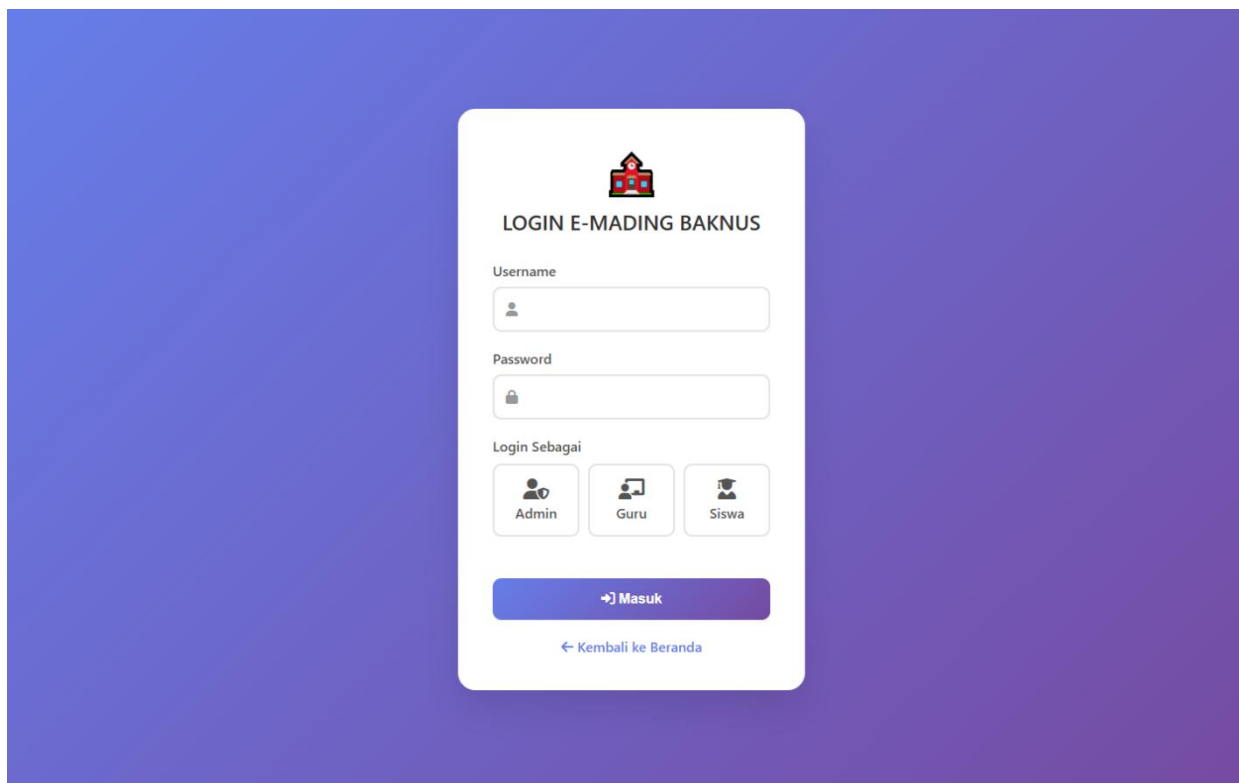
Tampilan Login
