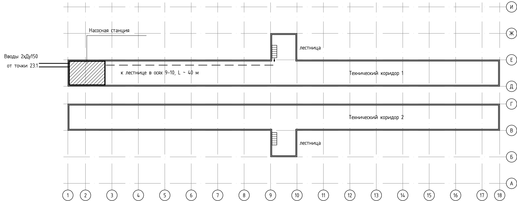
Схема расположения насосной станции М 1:500
