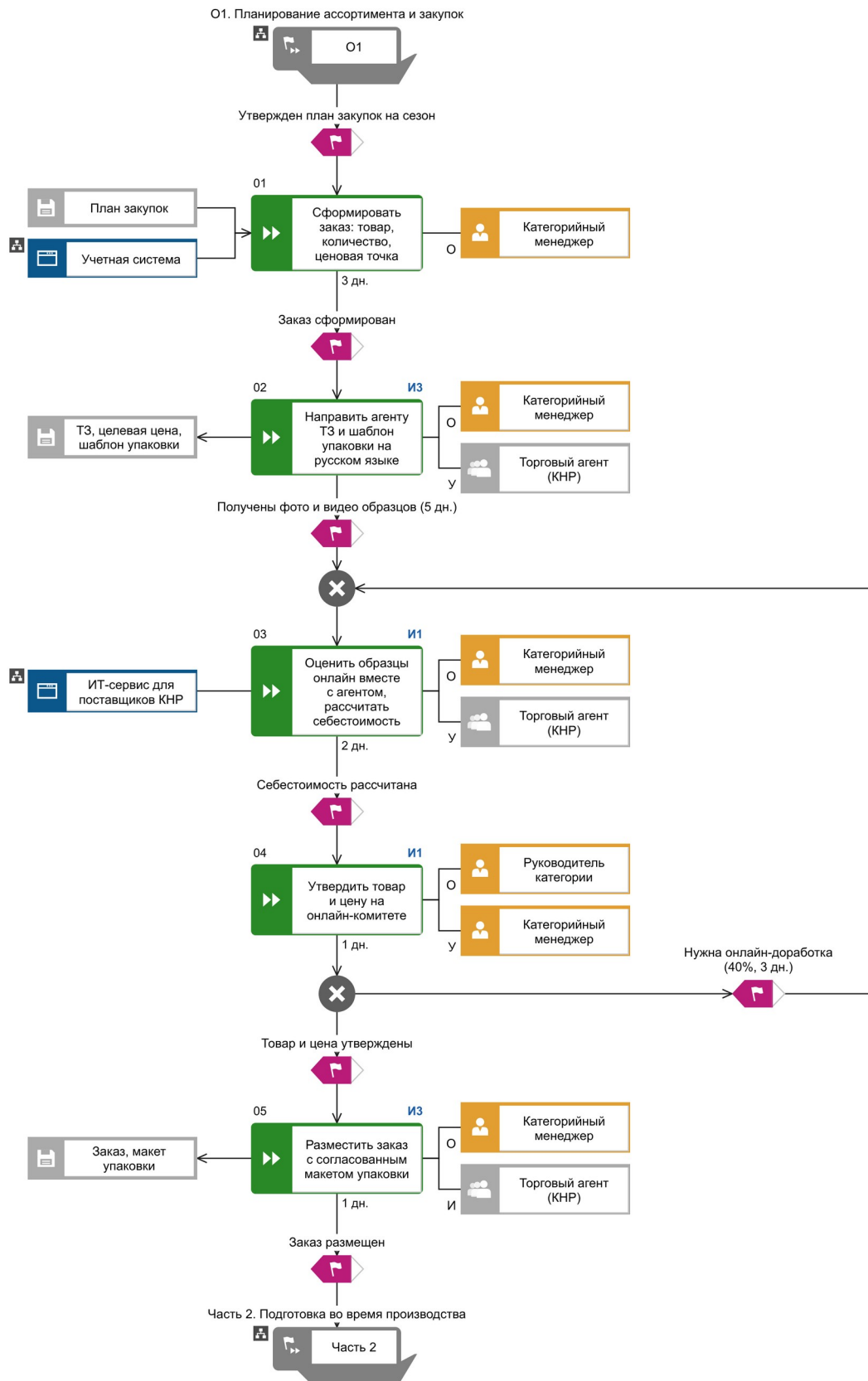
Рисунок 12 – Модель TO BE, часть 1: выбор товара и размещение заказа
