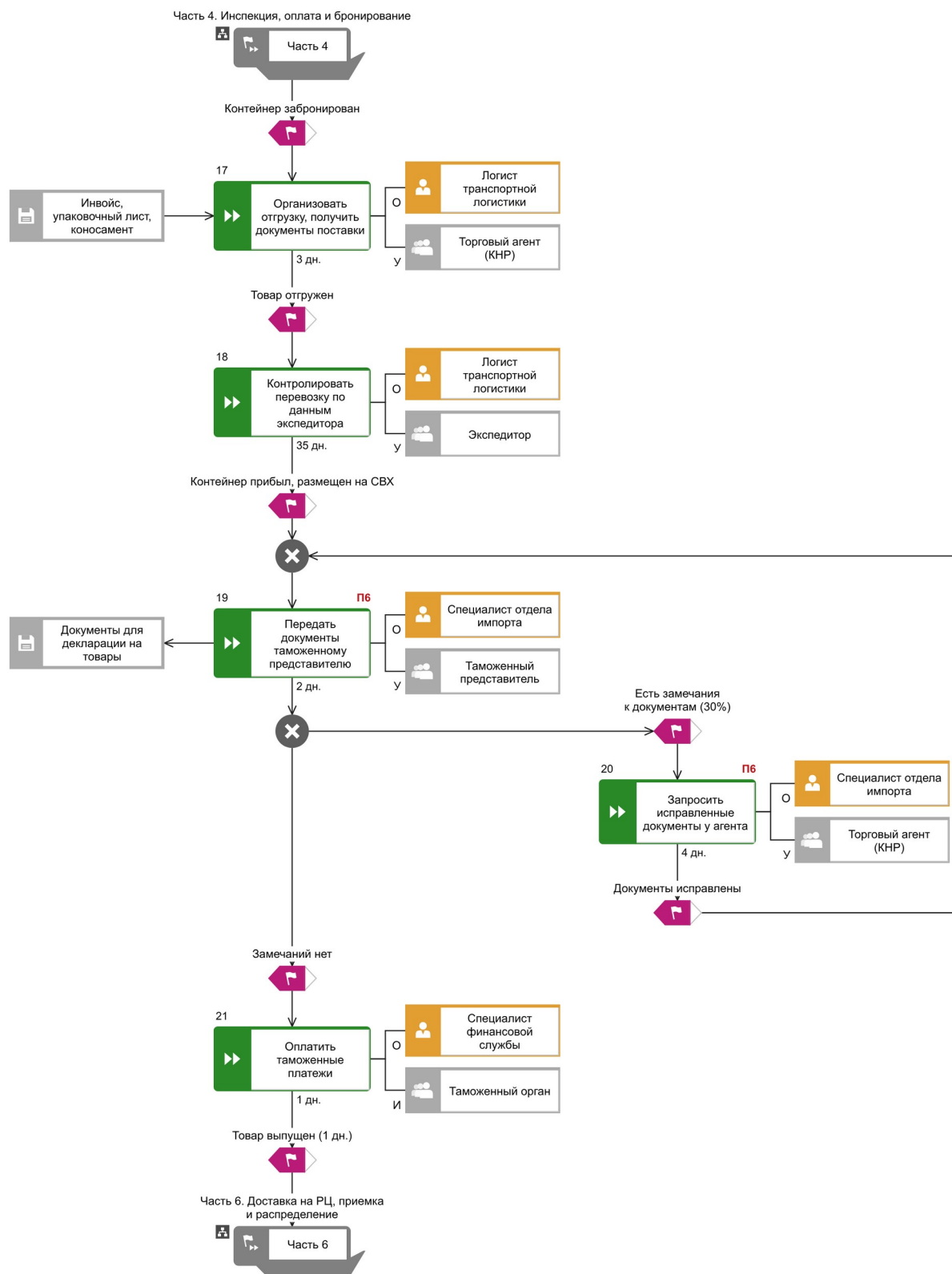
Рисунок 10 – Модель AS IS, часть 5: отгрузка, перевозка и таможенное оформление
