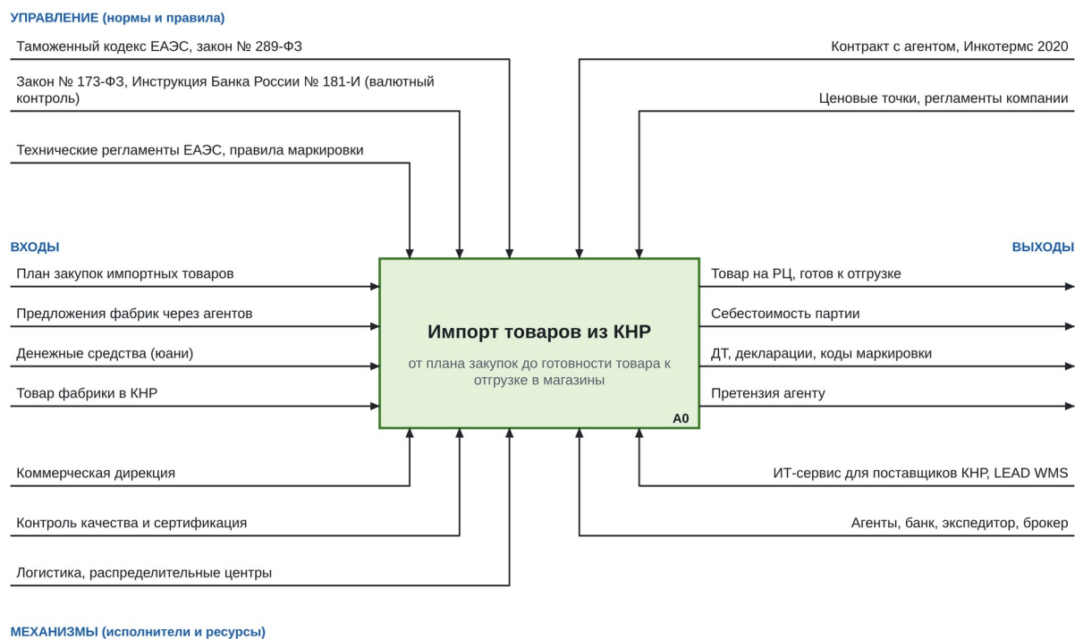
Рисунок 3 – Контекстная диаграмма процесса «Импорт товаров из КНР» (нотация IDEF0, диаграмма A-0)
