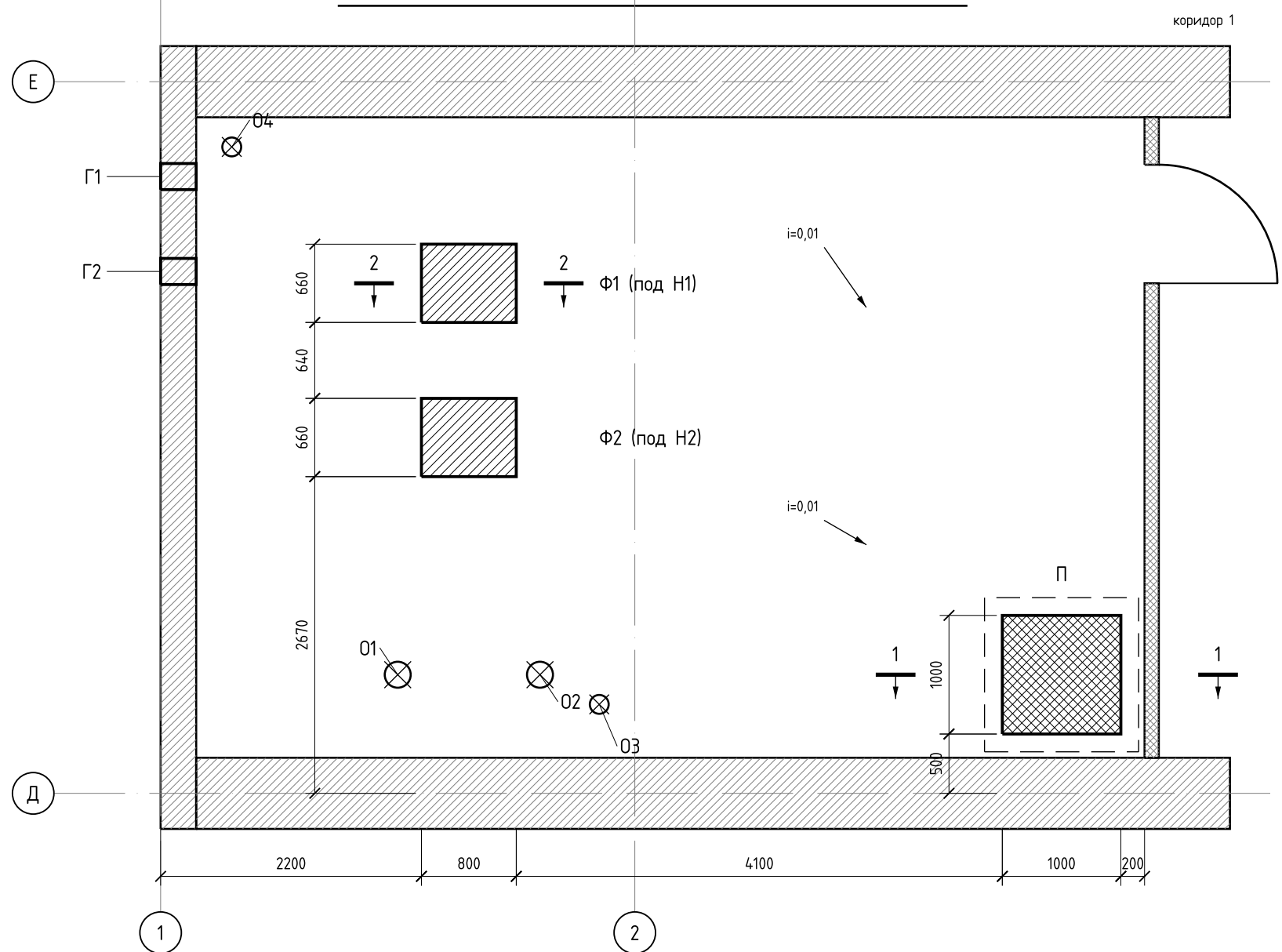
План насосной станции на отм. -2,200 (фрагмент) М 1:50
