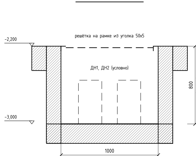
Разрез 1-1 М 1:20
