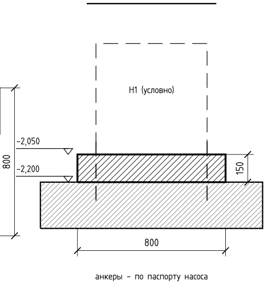
Разрез 2-2 М 1:20
