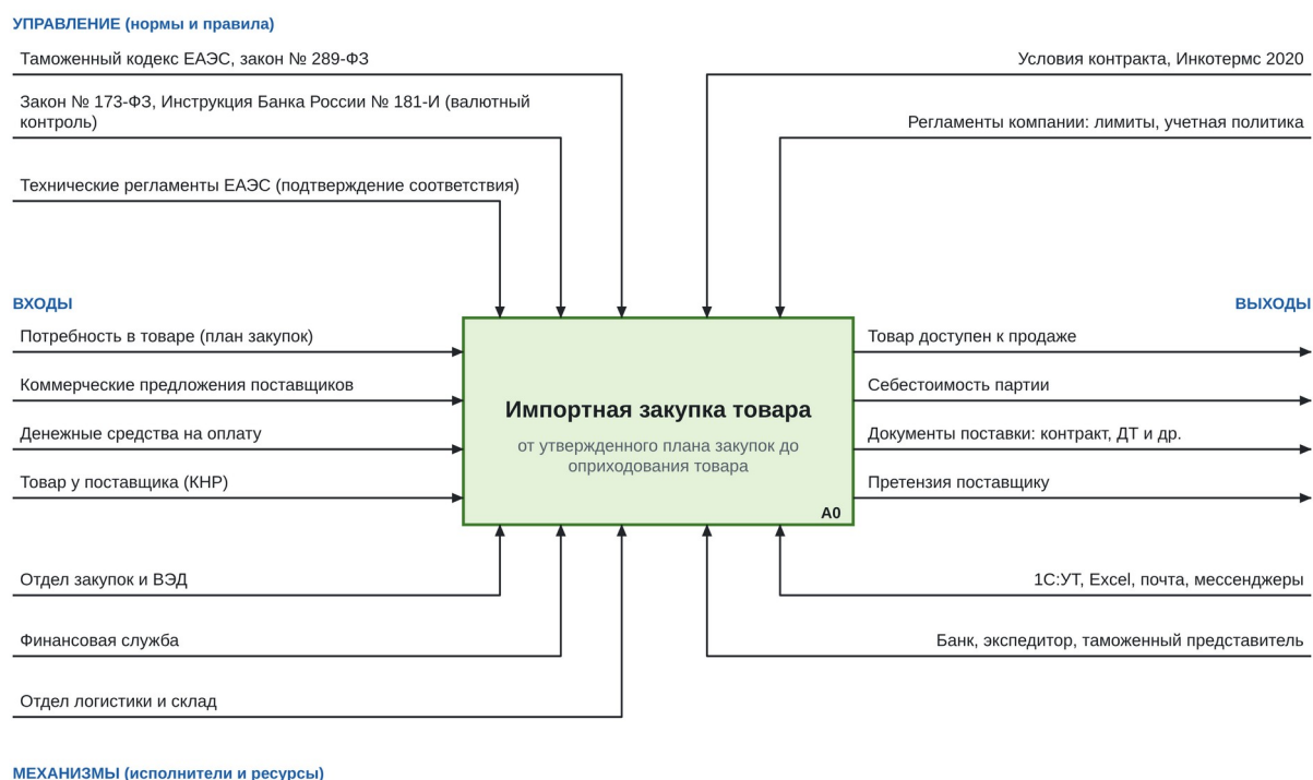
Рисунок 3 – Контекстная диаграмма процесса «Импортная закупка товара» (нотация IDEF0, диаграмма A-0)
