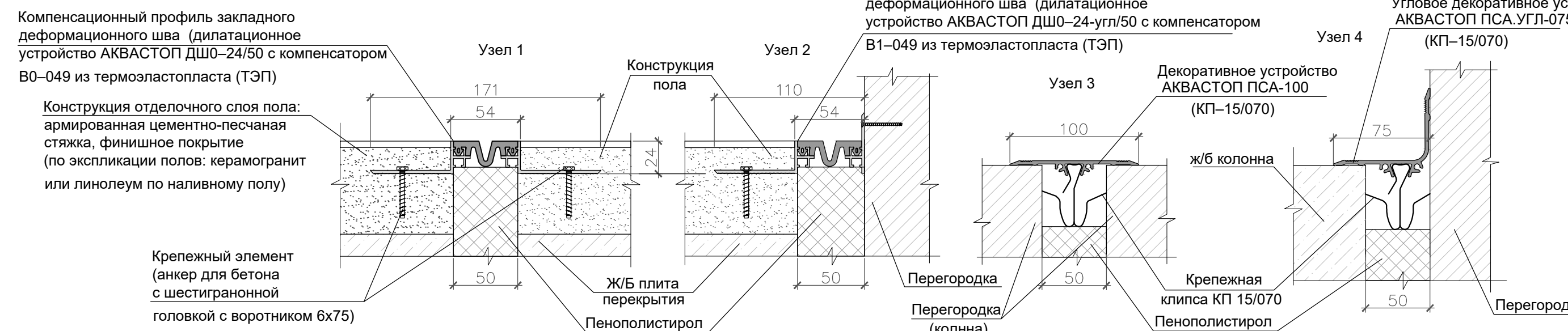
Узлы отделки деформационного шва по оси 7 (см. п.7)
