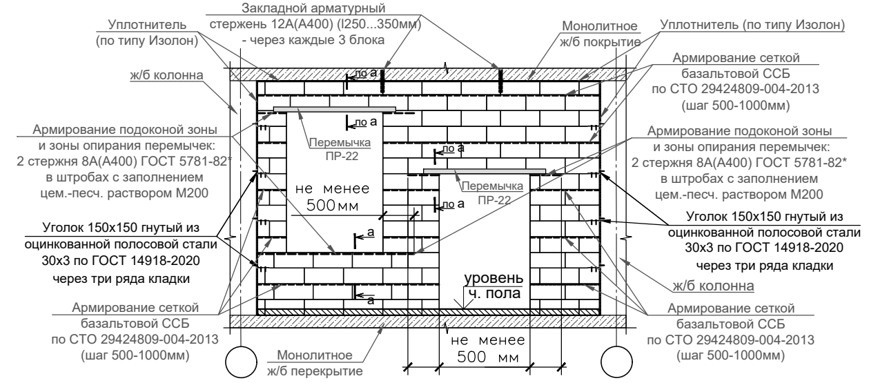
Схема примыкания к ж/б конструкциям и схема армирования наружных стен из газобетонных блоков.
