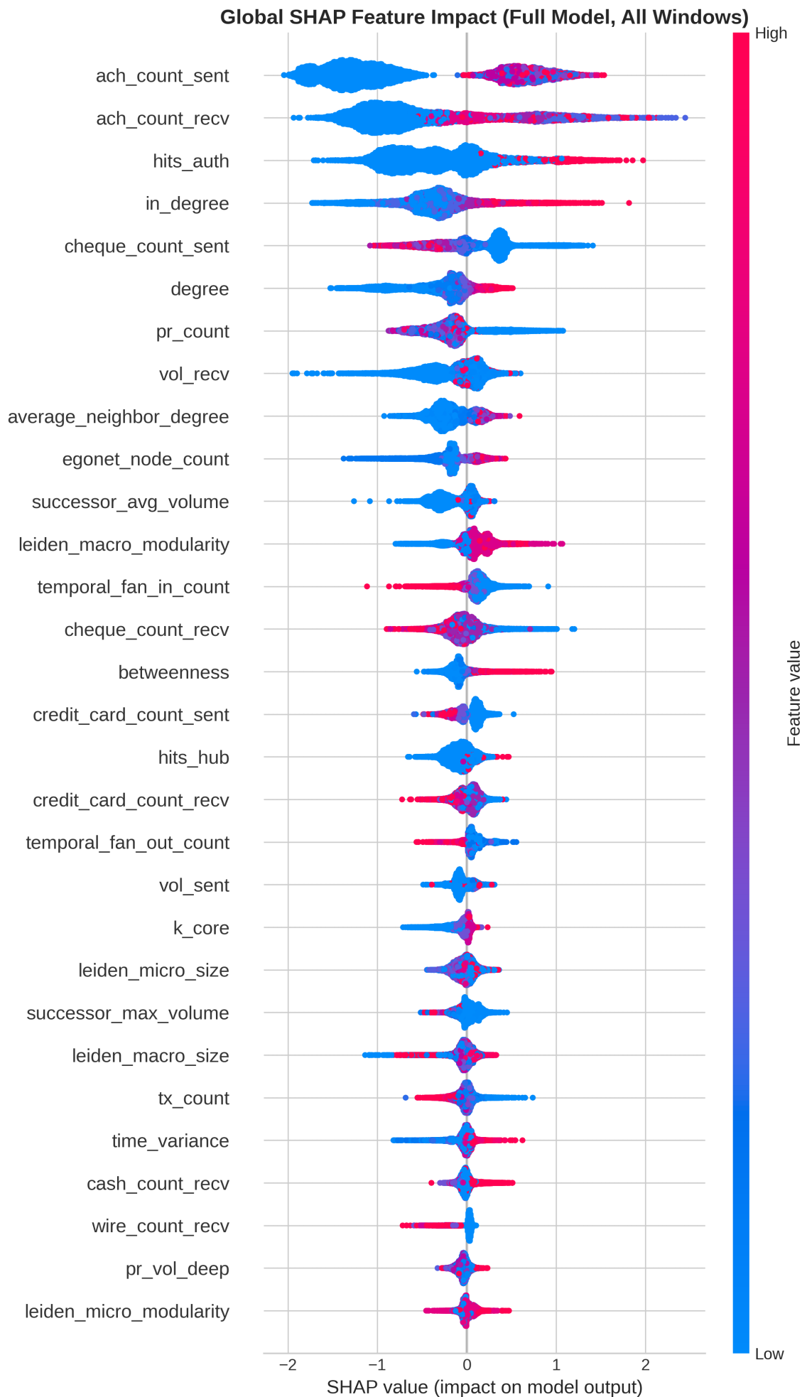
Figura 10 – Distribuição de valores SHAP para as principais features do modelo (HI Medium)
