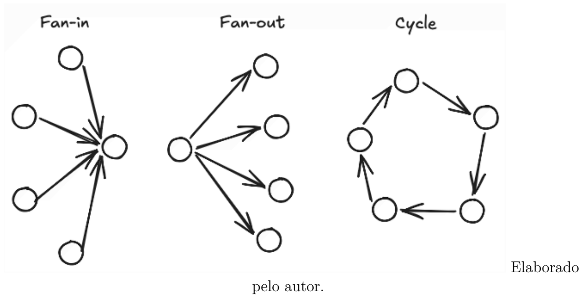
Figura 2 – Fan-in, Fan-out e Ciclo Direcionado em Grafos Financeiros
