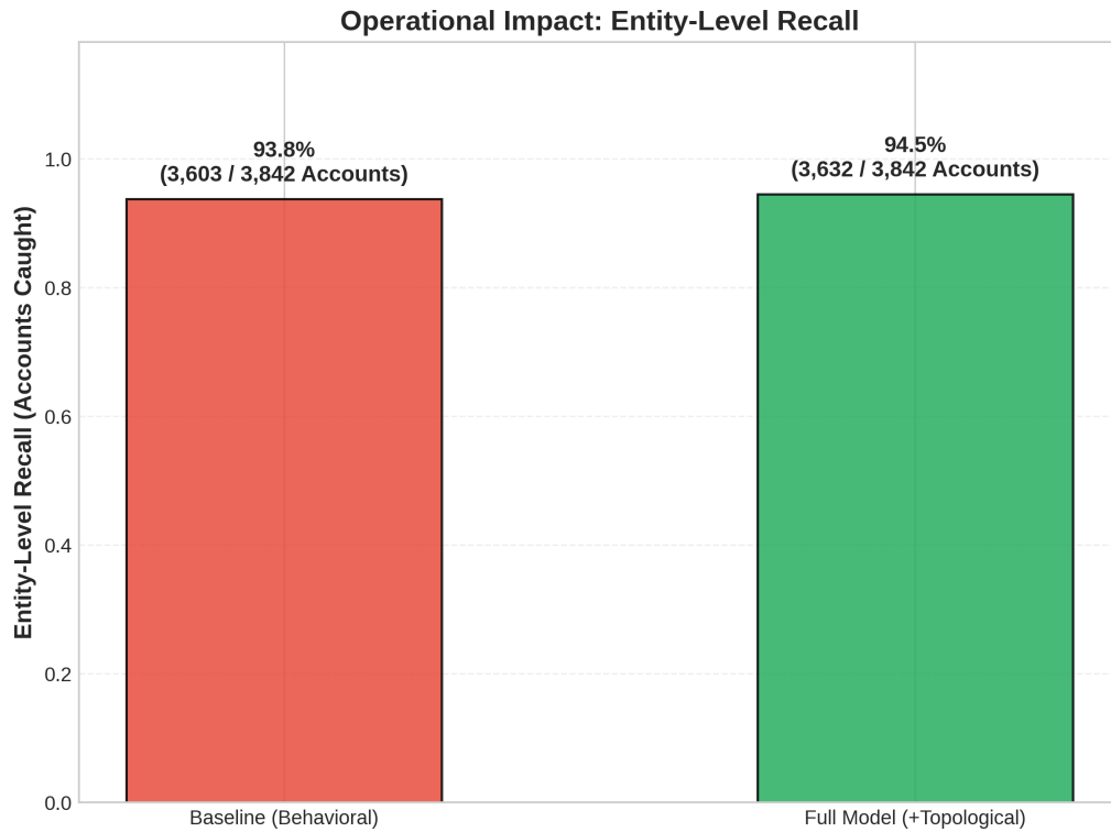
Figura 7 – Captura de entidades fraudulentas: Baseline vs Full Model (HI Small)
