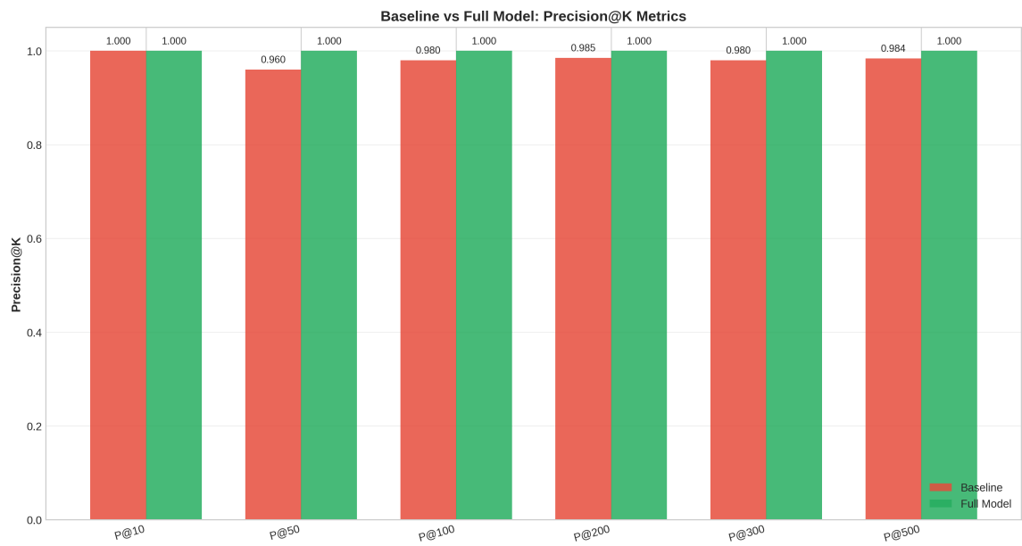
Figura 6 – Comparação de Precision@k entre os modelos Baseline e Full Model (HI Medium)
