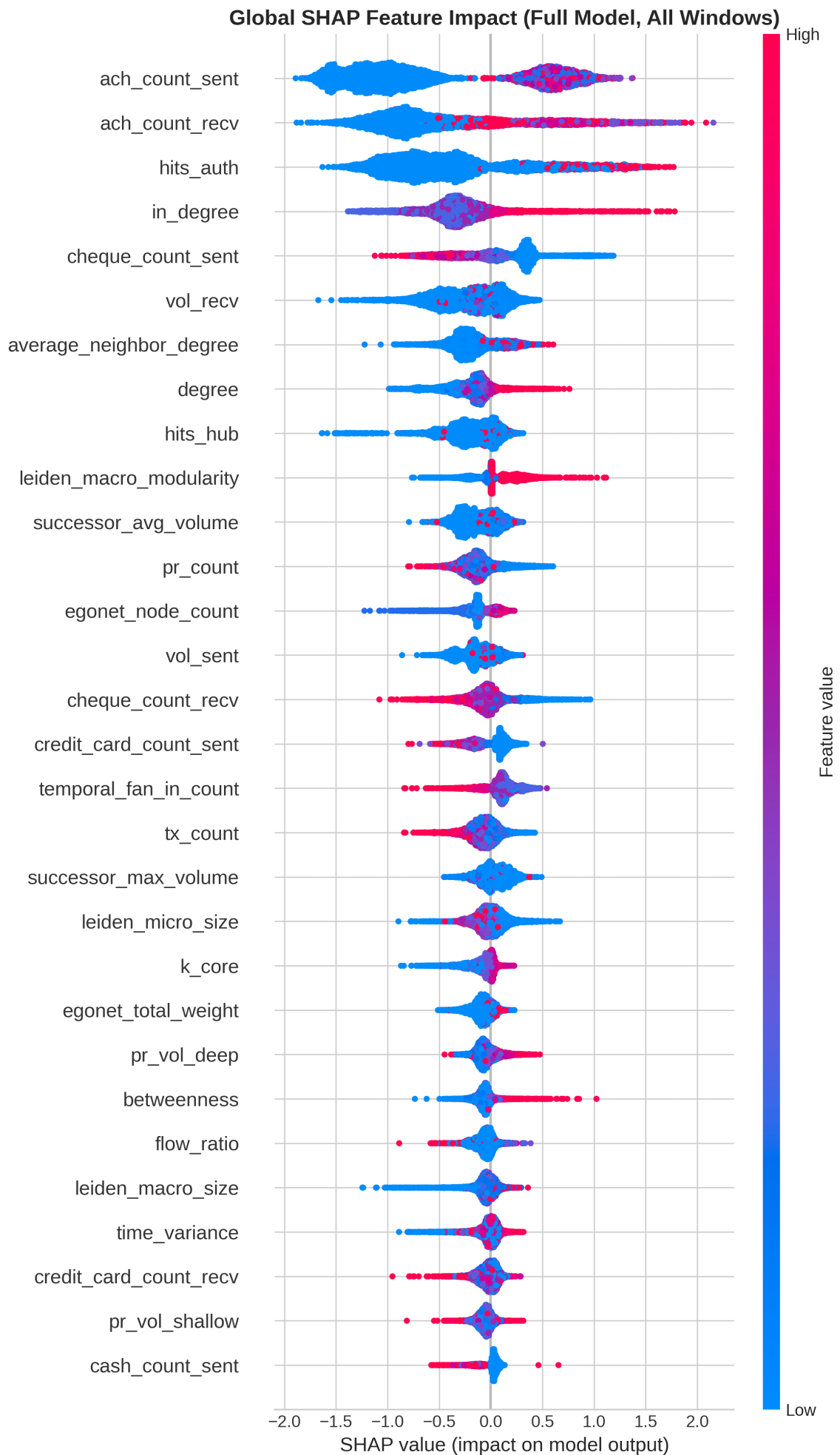
Figura 9 – Distribuição de valores SHAP para as principais features do modelo (HI Small)
