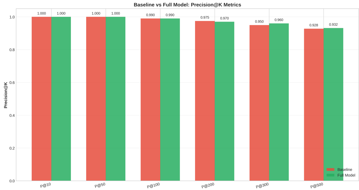
Figura 5 – Comparação de Precision@k entre os modelos Baseline e Full Model (HI Small)
