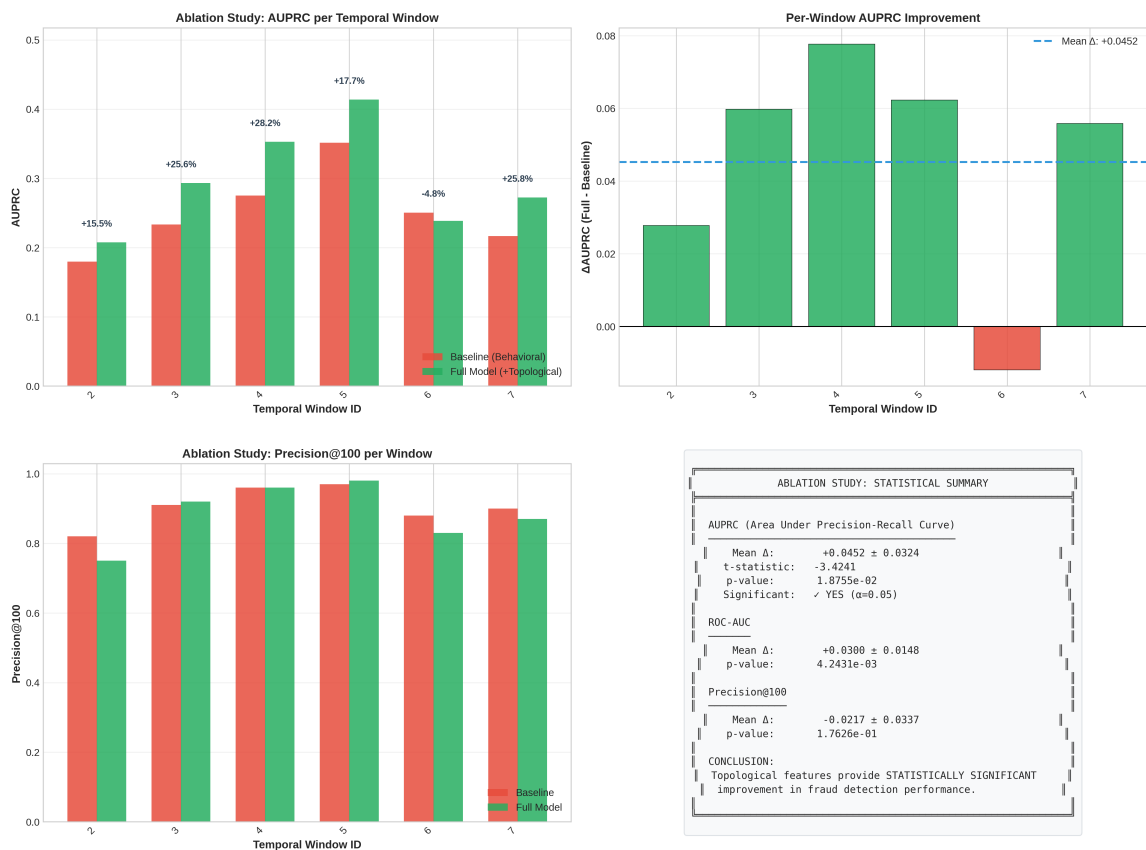
Figura 12 – Lift percentual por janela temporal e métrica de avaliação (HI Small)
