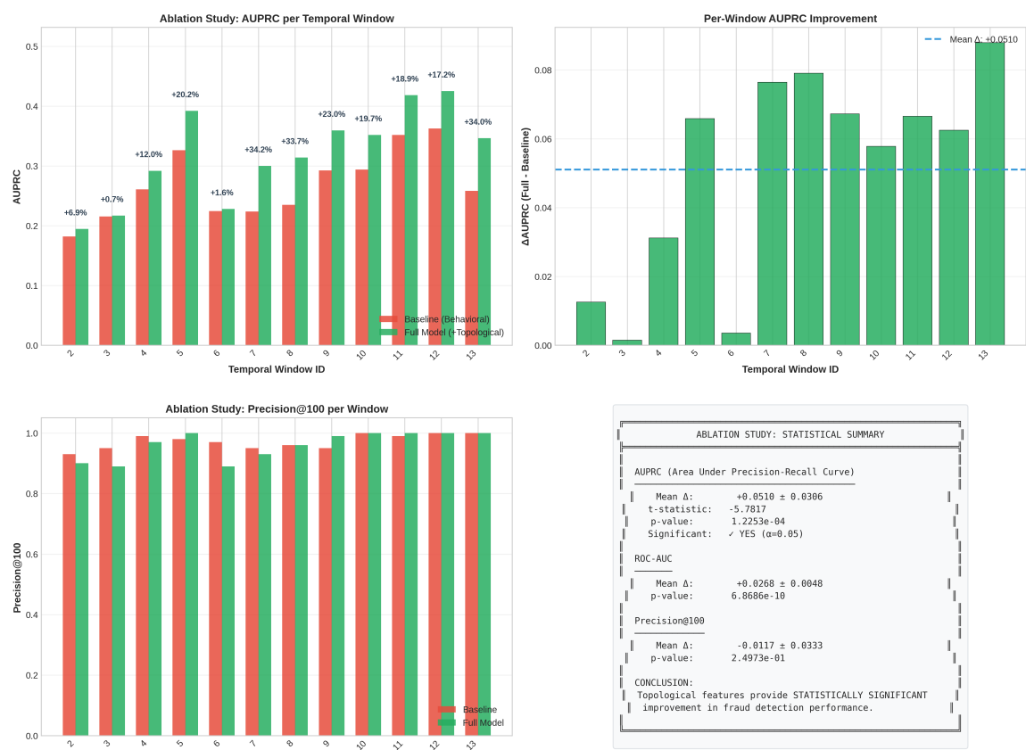
Figura 13 – Lift percentual por janela temporal e métrica de avaliação (HI Medium)
