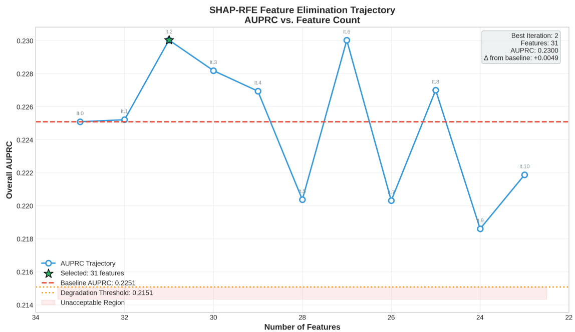
Figura 10 – Trajetória de degradação durante o processo SHAP-RFE (HI Small)
