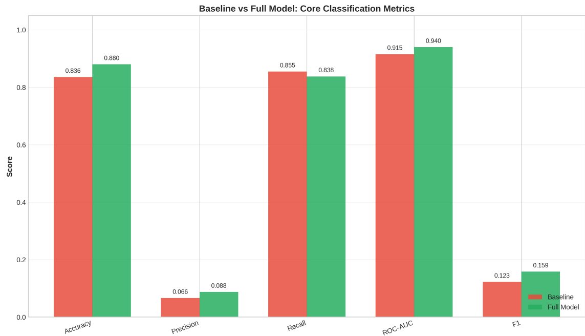
Figura 2 – Comparação de métricas entre os modelos Baseline e Full Model (HI Medium)
