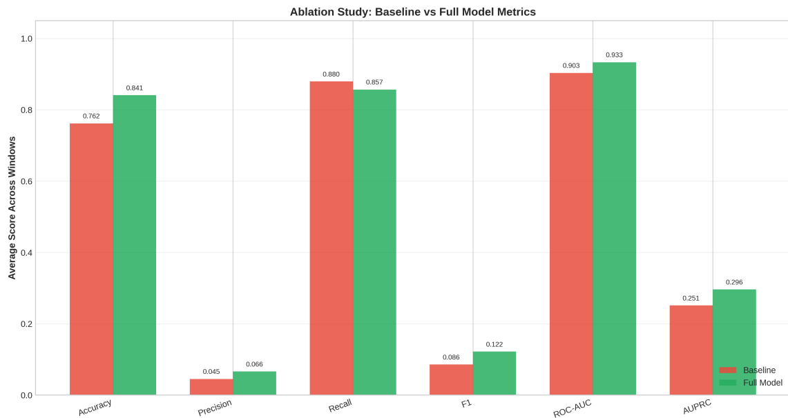
Figura 9 – Comparação estatística das métricas de ablação (HI Small)
