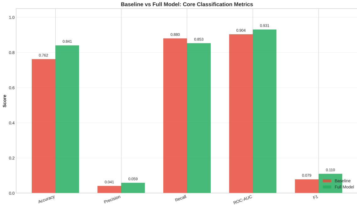
Figura 1 – Comparação de métricas entre os modelos Baseline e Full Model (HI Small)
