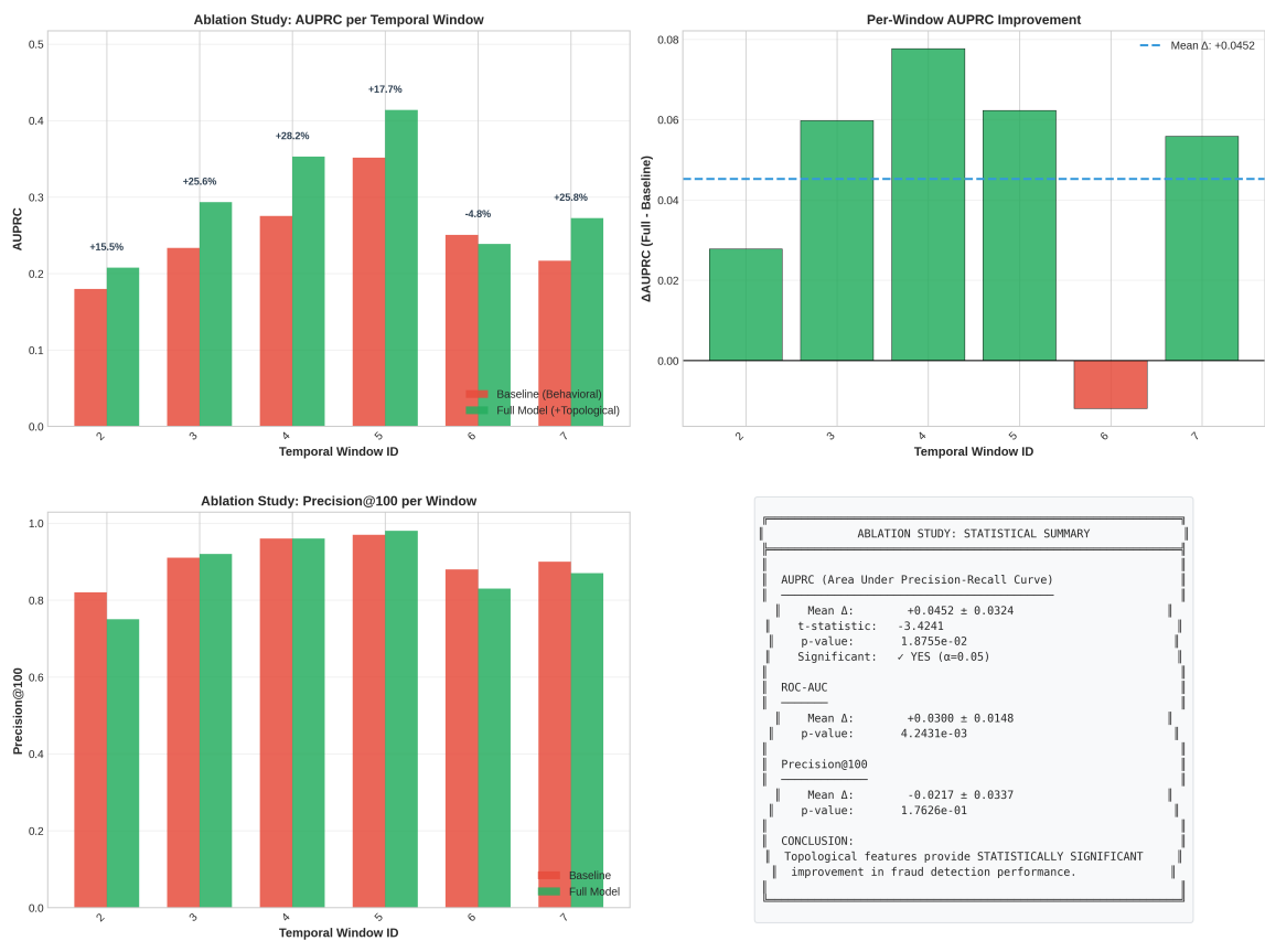
Figura 10 – Lift percentual por janela temporal e métrica de avaliação (HI Small)
