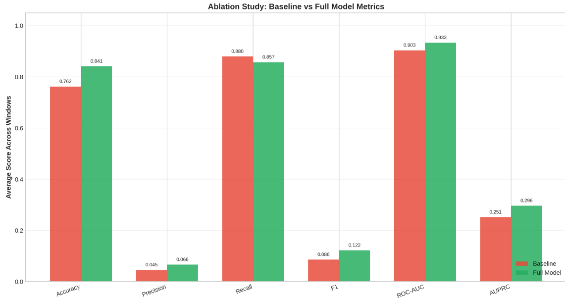
Figura 2 – Comparação de métricas entre os modelos Baseline e Full Model (HI Small)
