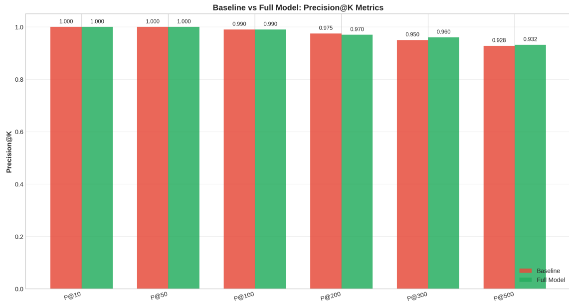
Figura 4 – Comparação de Precision@k entre os modelos Baseline e Full Model (HI Small)
