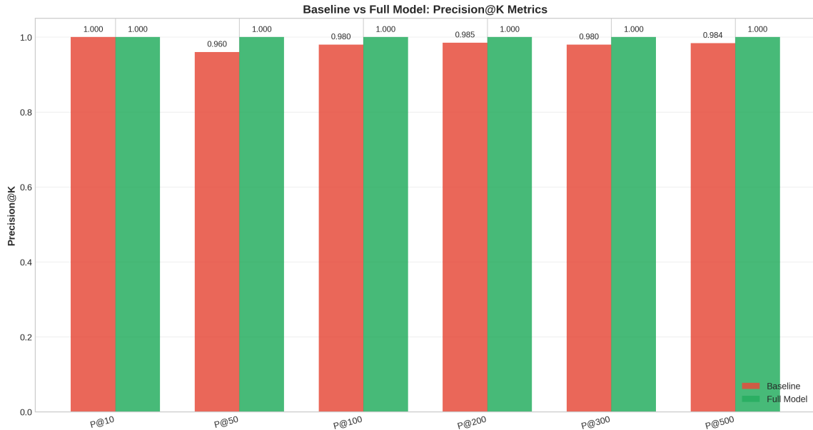
Figura 5 – Comparação de Precision@k entre os modelos Baseline e Full Model (HI Medium)
