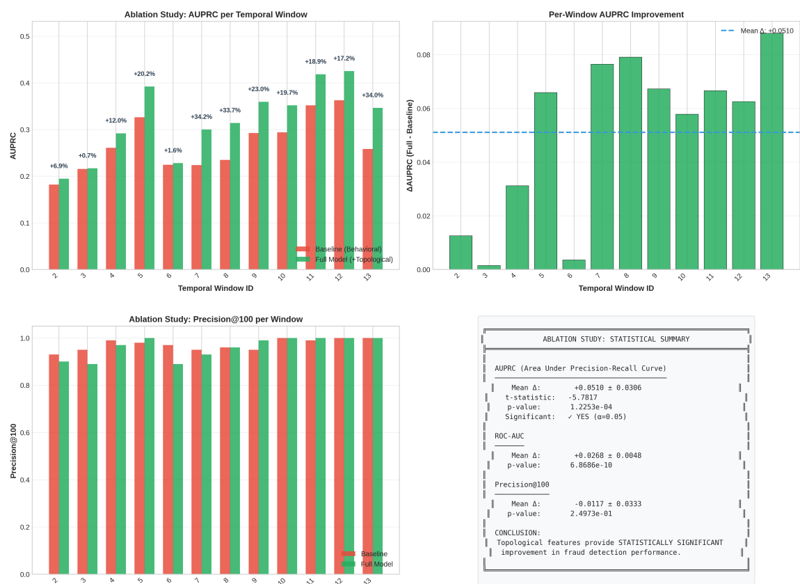
Figura 11 – Lift percentual por janela temporal e métrica de avaliação (HI Medium)
