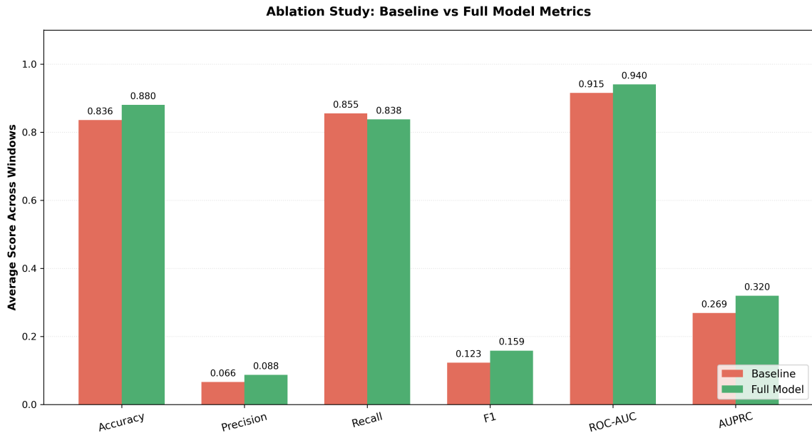
Figura 3 – Comparação de métricas entre os modelos Baseline e Full Model (HI Medium)
