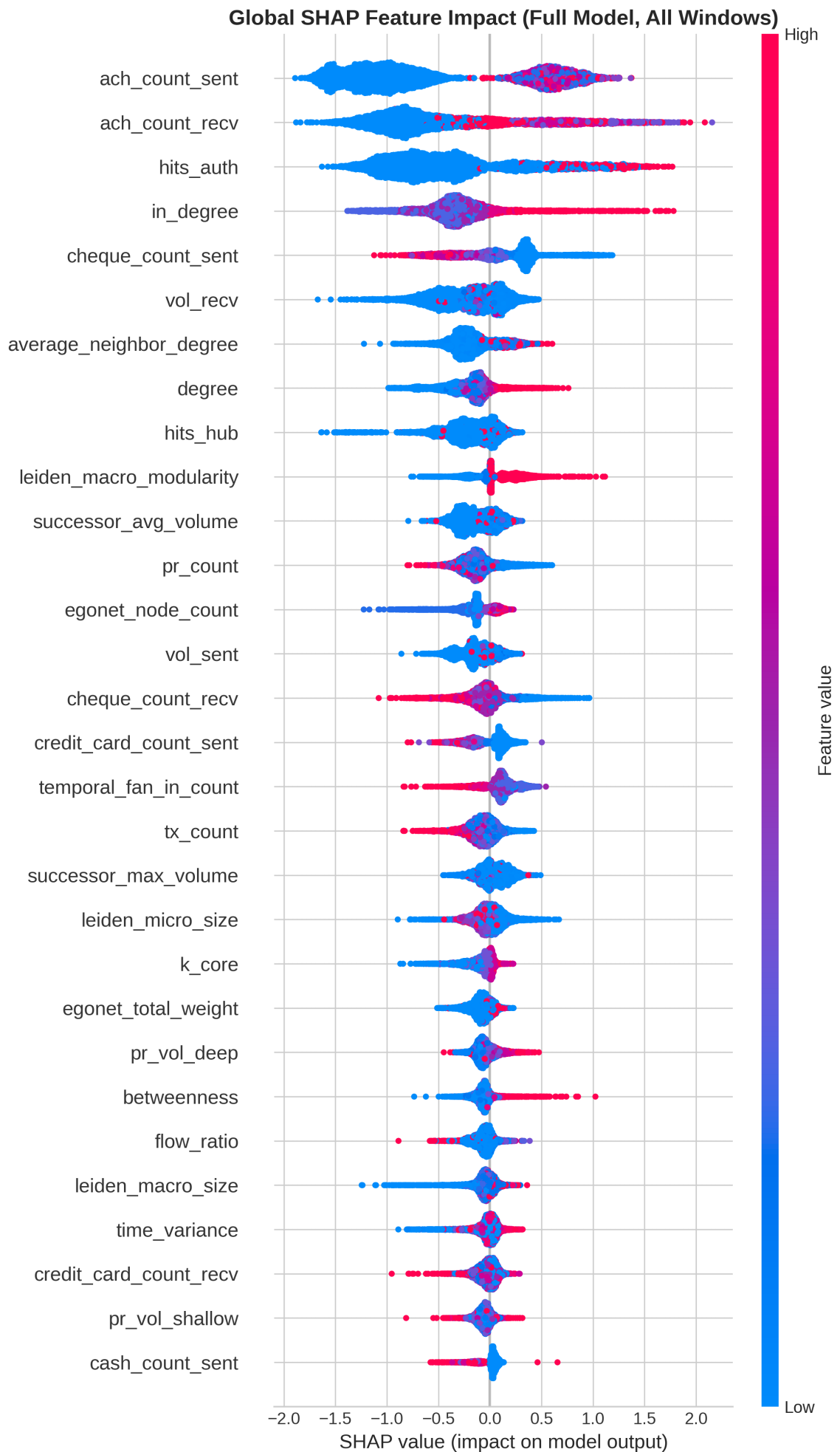
Figura 8 – Distribuição de valores SHAP para as principais features do modelo (HI Small)
