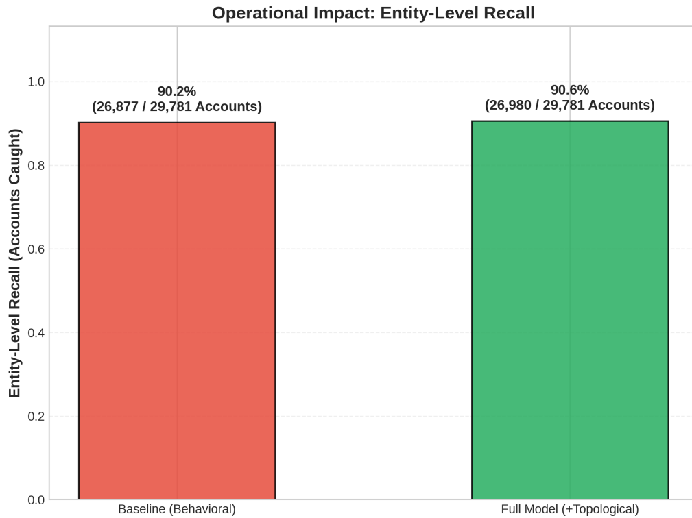
Figura 7 – Captura de entidades fraudulentas: Baseline vs Full Model (HI Medium)
