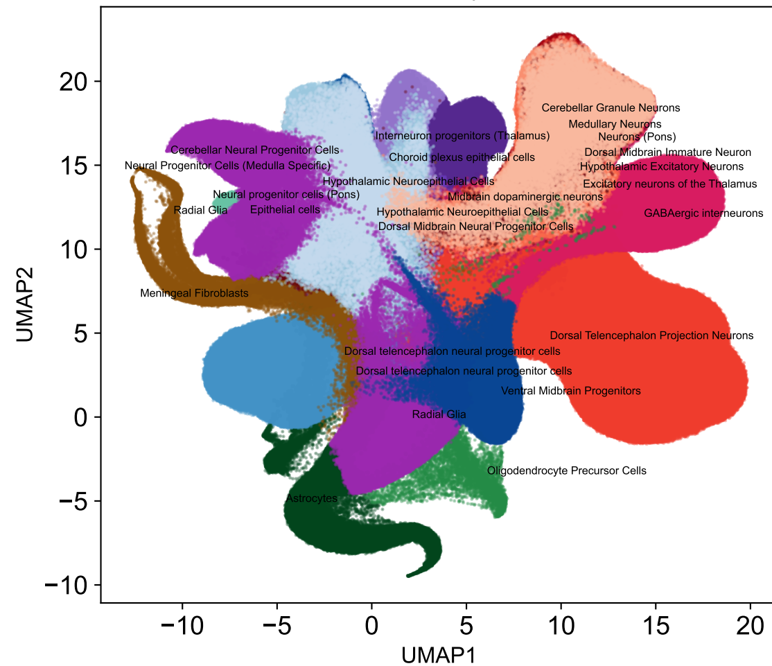
GPTCelltype
