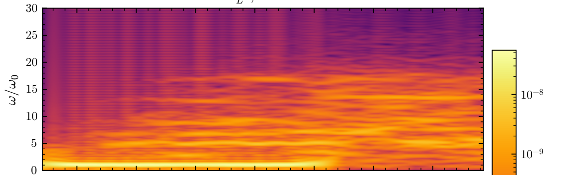
(b) I_L^{S_\alpha}, \alpha = y
