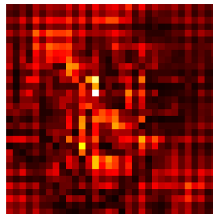
ViT Gradient
