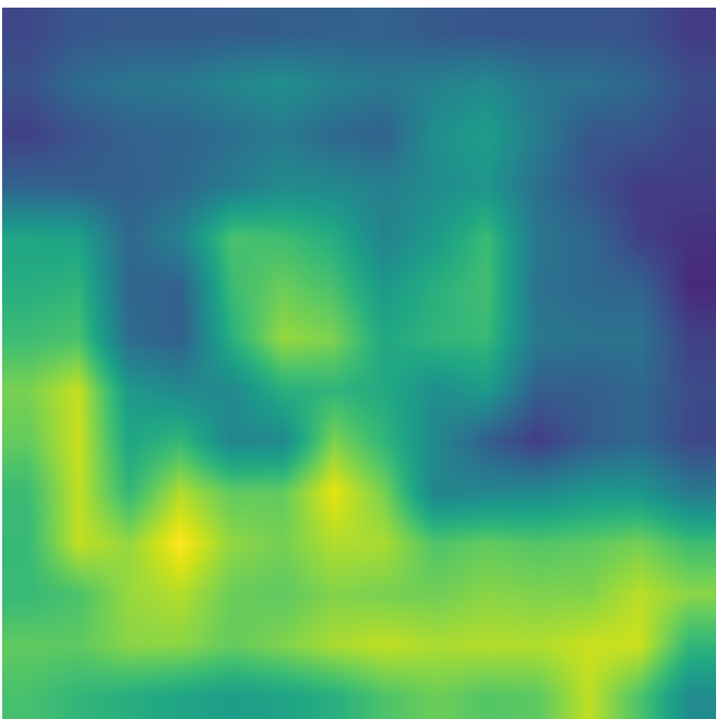
Layer 6 Clean
