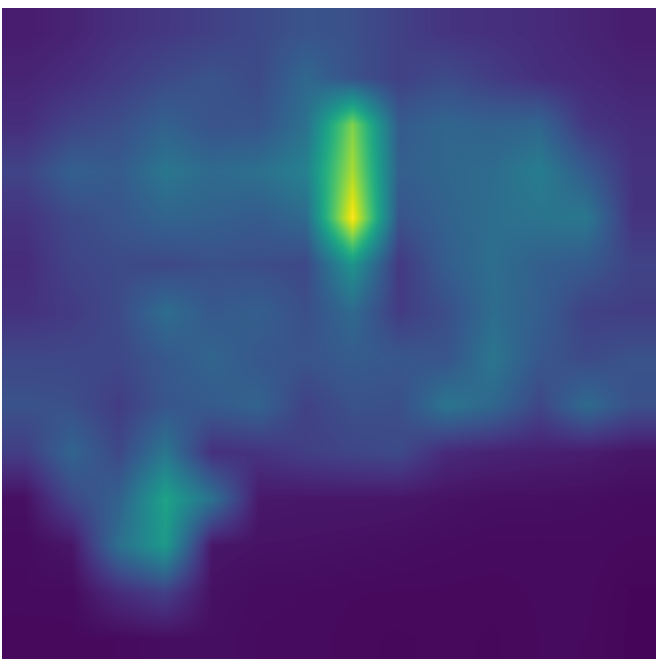
Layer 12 Clean
