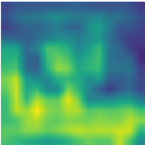
Layer 6 Clean
