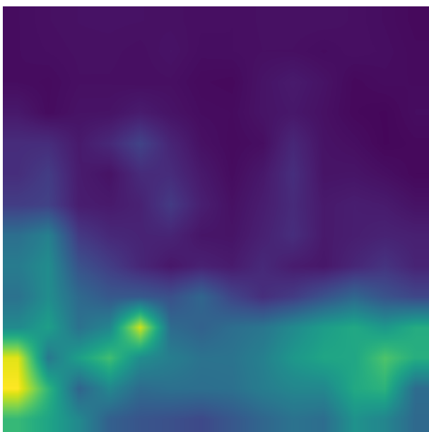
Layer 12 Clean
