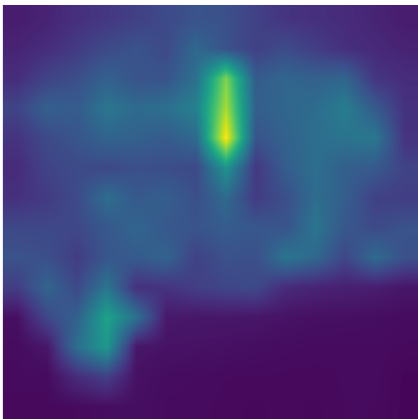
Layer 12 Clean
