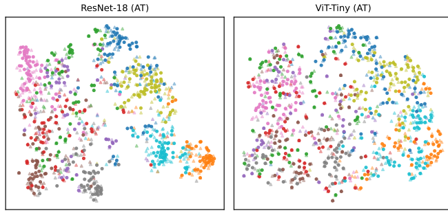
Şekil 9: Temiz örnekler (daireler) ve her modelin kendi beyaz kutu PGD-10 çekişmeli örnekleri (üçgenler) için sondan bir önceki katman öznelitliklerinin gösterim amaçlı t-SNE gömmesi; ResNet-18 (sol) ve ViT-Tiny (sağ). t-SNE yalnızca yönlendirme içindir; nicel karşılaştırma metinedir.
