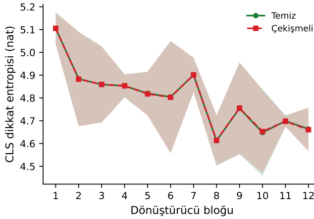
Şekil 8: Temiz ve çekişmeli girdiler için CLS dikkat dağılımının katman başına entropisi; koşum başına n = 1000 örnek, üç koşum ortalaması ve \pm 1 std bandı. Dikkat haritalarının kendisi Şekil 7’te verilmektedir.
