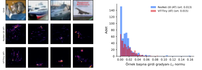
(a) Girdi alanı görselleştirilmesi (b) Örnek başına gradyan L_2 norm dağılımı
