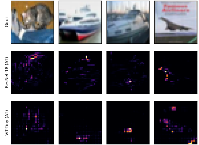
Şekil 6: Aynı girdiler üzerinde CNN ve ViT gradyan enerjisi haritalarının karşılaştırması. Farklar Tablo VI’teki seyreklik ölçüleriyle nicelenir; Tablo VII, görünür yapının mekânsal kümelenme farkına karşılık gelmediğini gösterir.
