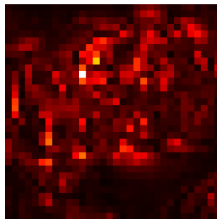
CNN Gradient
