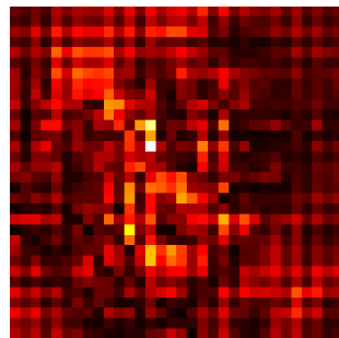
ViT Gradient
