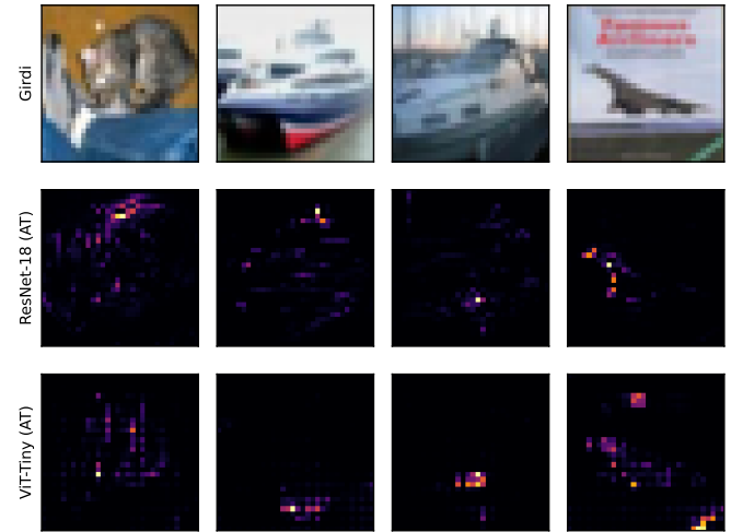
Şekil 6: Aynı girdiler üzerinde CNN ve ViT gradyan enerji haritalarının karşılaştırması. Farklar Tablo VII’teki seyreklik ölçüleriyle nicelenir; Tablo VIII, görünür yapının mekânsal kümelenme farkına karşılık gelmediğini gösterir.
