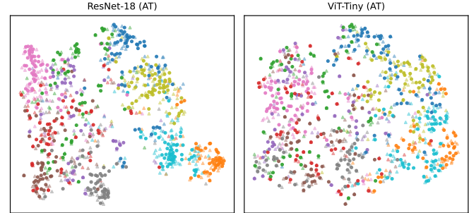
Şekil 9: Temiz örnekler (daireler) ve her modelin kendi beyaz kutu PGD-10 çekışmeli örnekleri (üçgenler) için sondan bir önceki katman özniteliklerinin gösterim amaçlı t-SNE gömmesi; ResNet-18 (sol) ve ViT-Tiny (sağ). t-SNE yalnızca yönlendirme içindir; nicel karşılaştırma metinedir.
