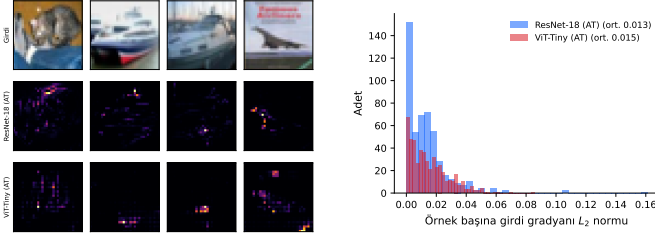
(a) Gradyan alanı görselleştirilmesi
