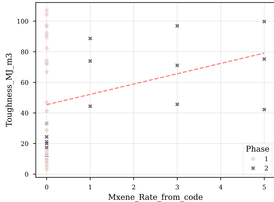
Toughness vs Mxene_Rate_from_code
